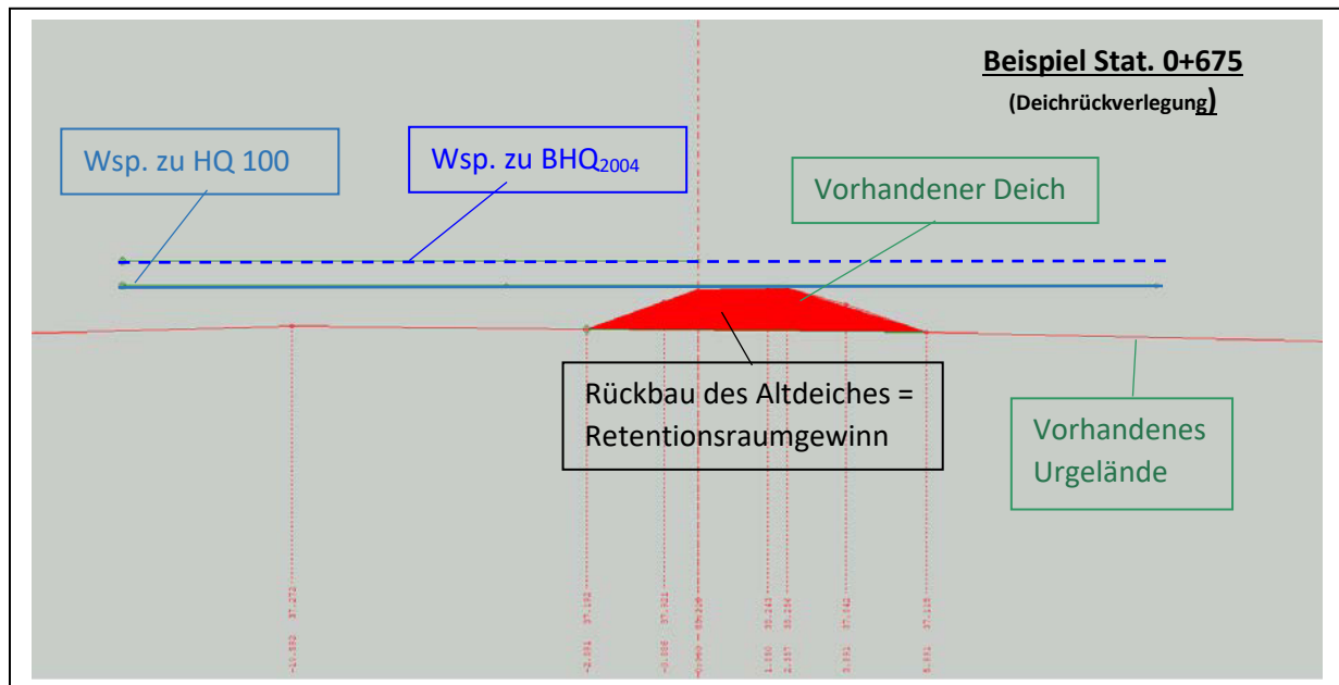
Beispiel: Berechnung des Retentionsraumgewinnes durch Altdeichrückbau
