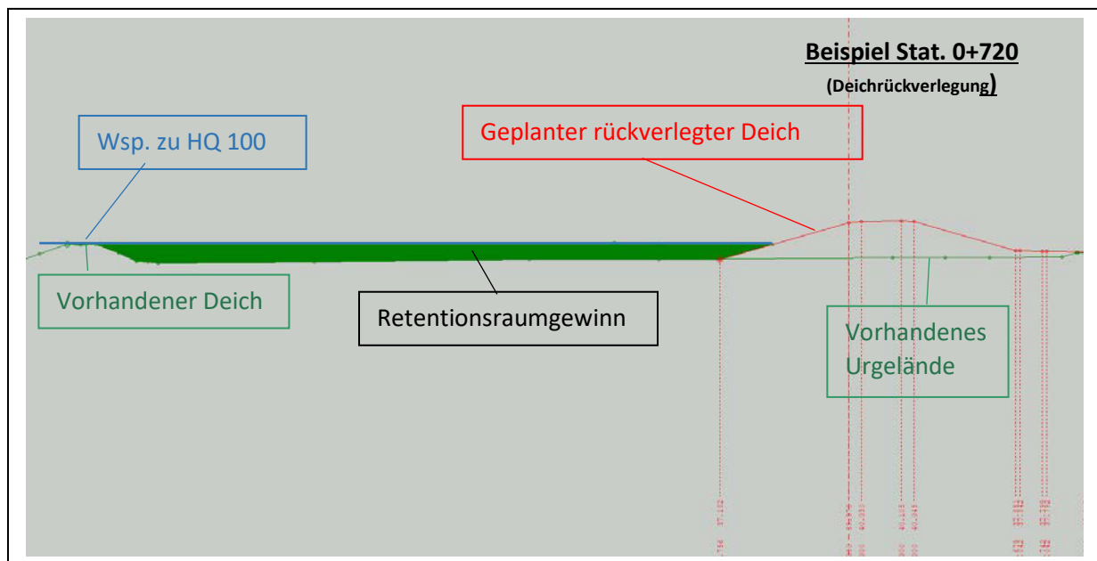
Beispiel: Berechnung des Retentionsraumgewinnes
