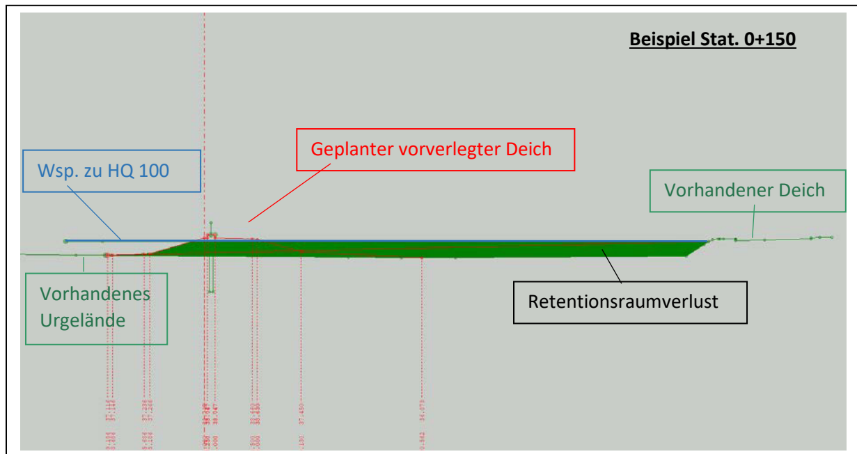
Beispiel: Berechnung des Retentionsraumverlustes
