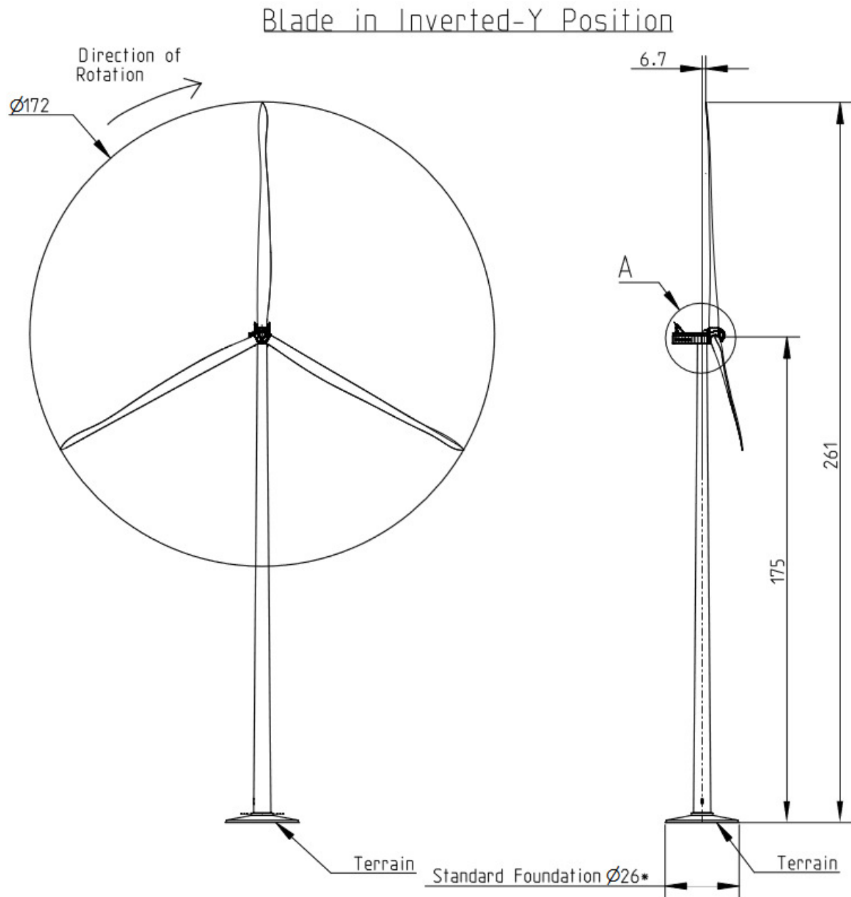
Abbildung 1: Übersichtszeichnung einer Vestas V172-7.2 mit 175 m Nabenhöhe (Quelle: VestasOnline)
