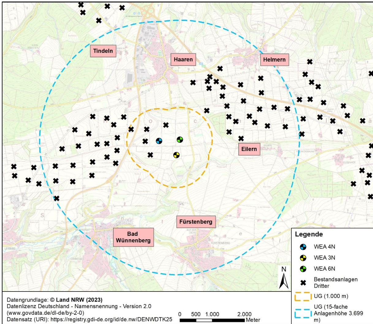
Abbildung 1 Lage der geplanten WEA-Standorte und der Bestands-Anlagen, sowie Darstellung der Untersuchungsgebiete
