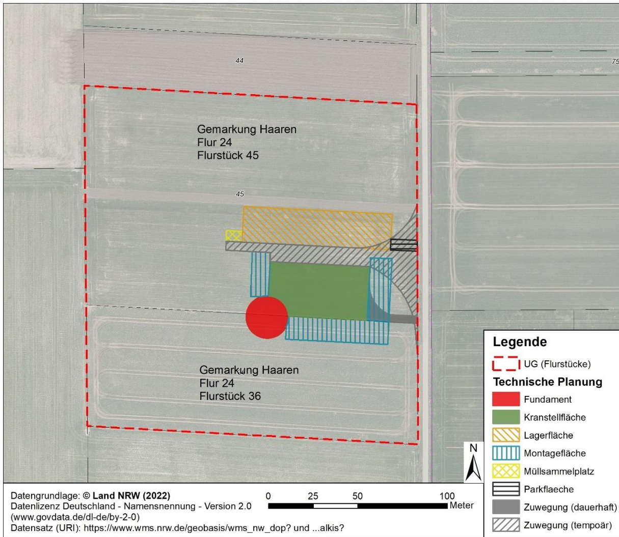
Abbildung 3 Erschließung und technische Planung von WEA 4N
