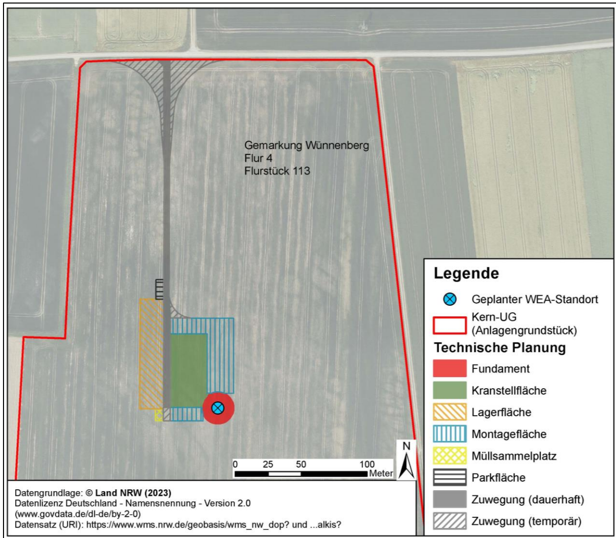
Abbildung 2 Erschließung und technische Planung von WEA 3N
