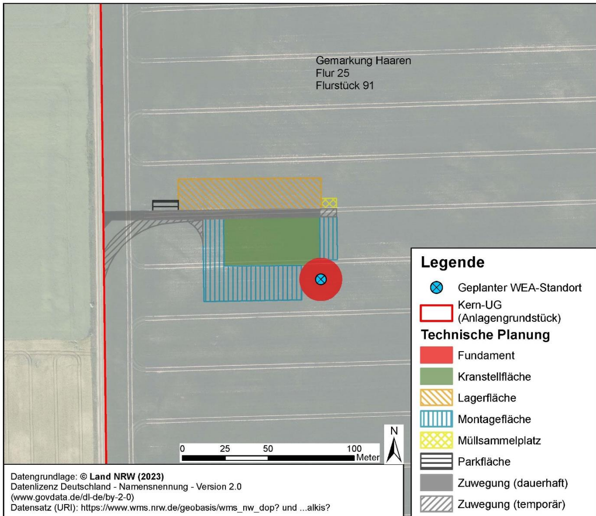
Abbildung 4 Erschließung und technische Planung von WEA 6N
