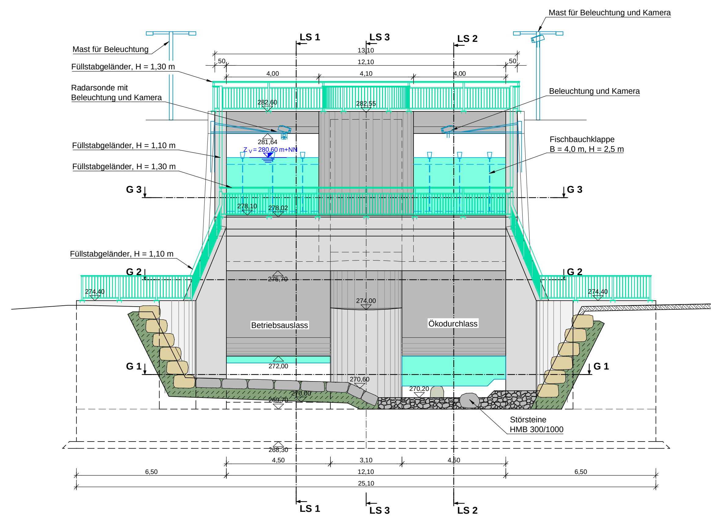
Ansicht Einlauf
