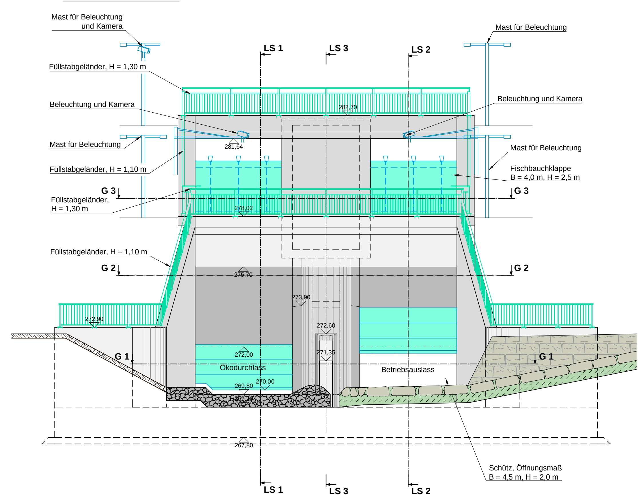
Ansicht Auslauf
