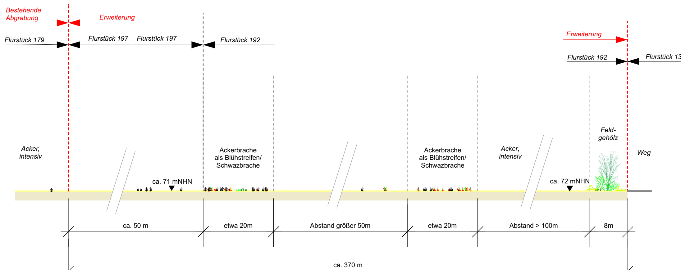
Schematisches Profil B Gestaltung
