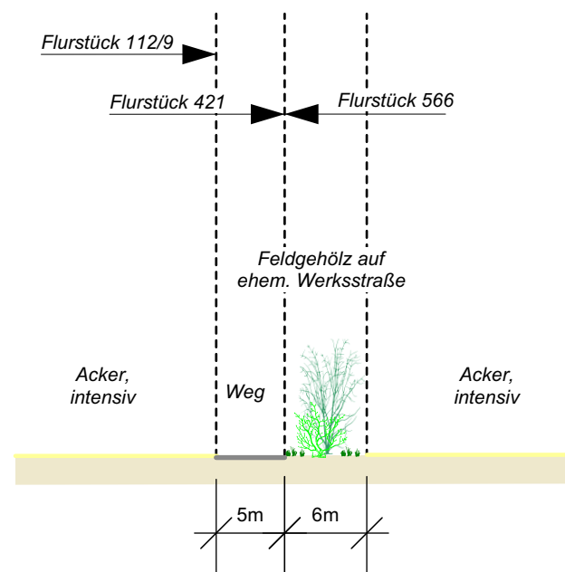
Schematisches Profil Gestaltung Zufahrt Südost M = 1:500
