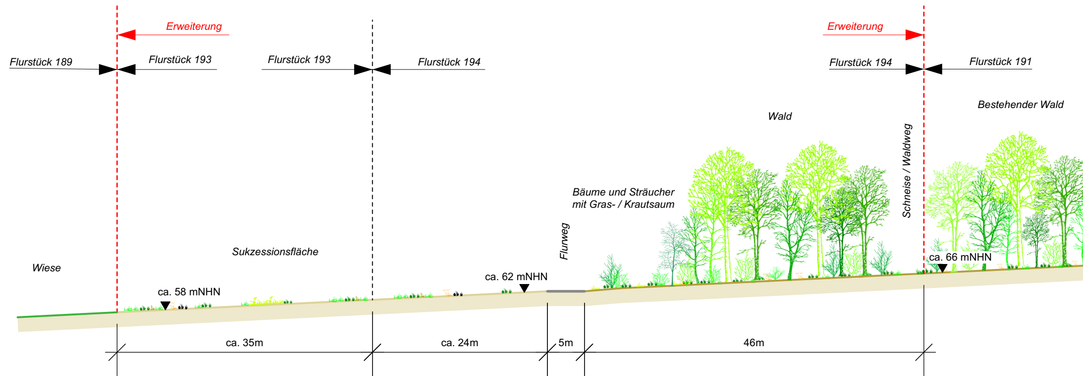
Schematisches Profil A Gestaltung
