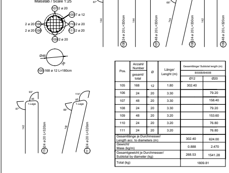
Schnitt / Section B-B Maßstab / Scale 1:25
