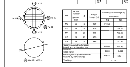
Schnitt / Section B-B Maßstab / Scale 1:25
