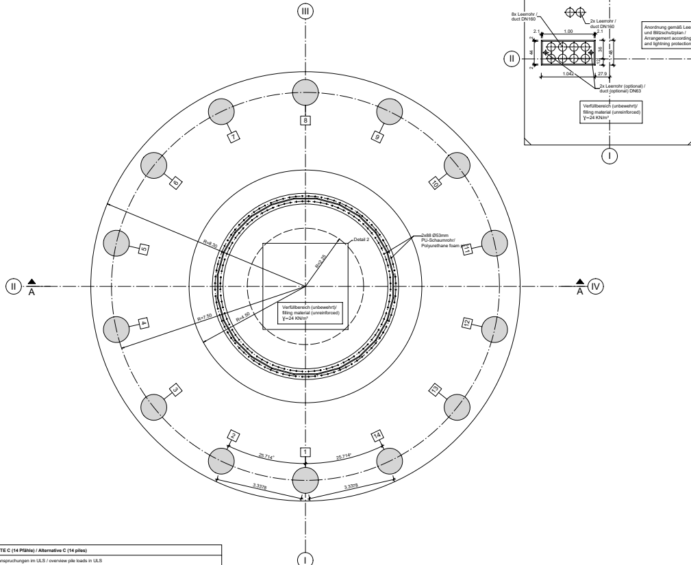
Draufsicht Fundament / Top view foundation Variante / option C
