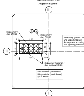
Detail 2 Maßstab / Scale 1:25
