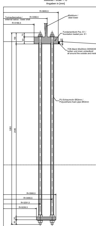
Detail 1 Maßstab / Scale 1:10
