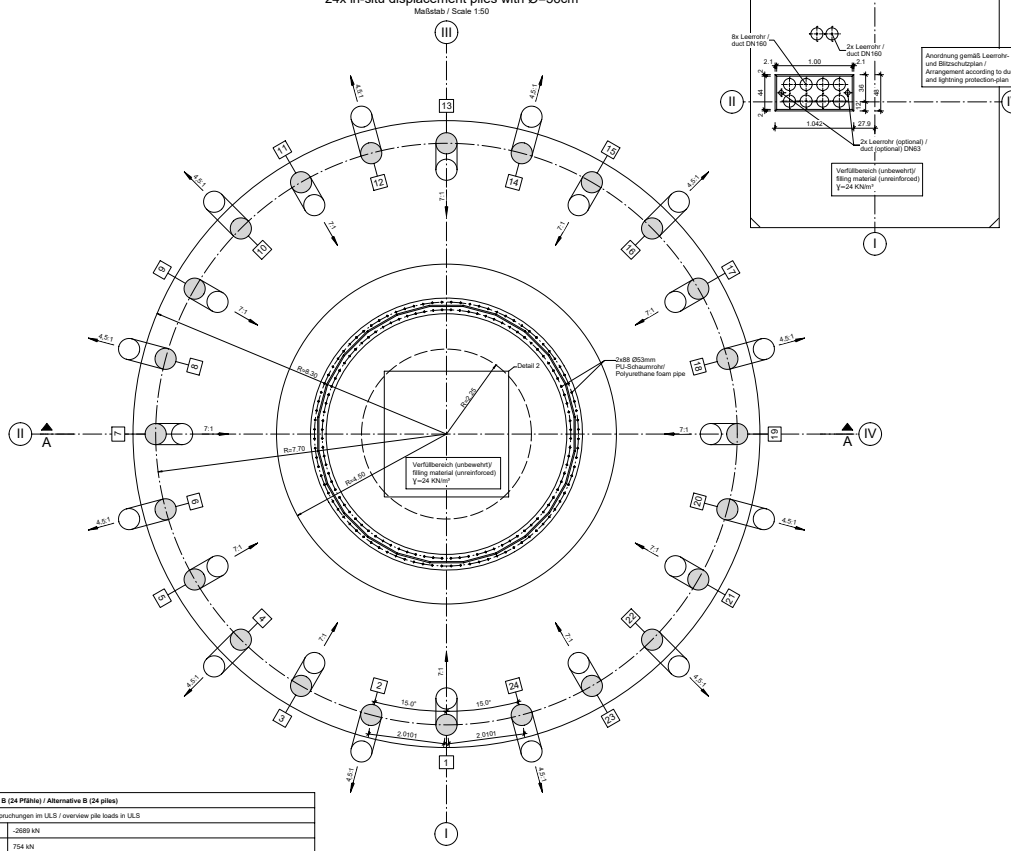
Draufsicht Fundament / Top view foundation
