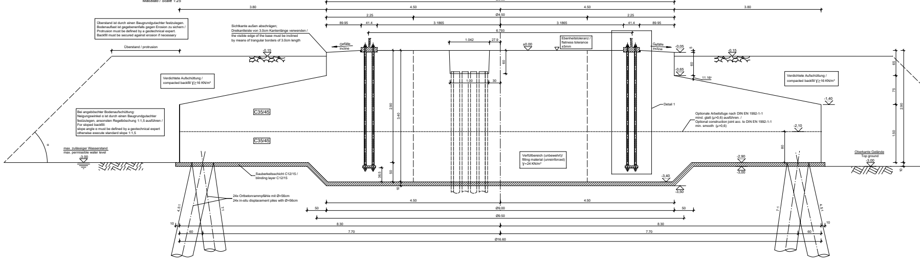
Detail 2 Maßstab / Scale 1:25 Angaben in [mm]
