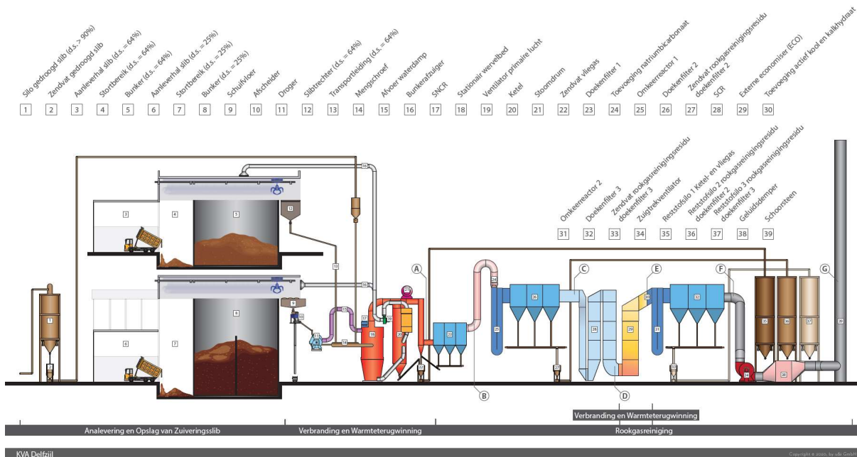
Figuur 6 Schematisch overzicht SVI (in Bijlage B is de vergrote weergave te vinden)
