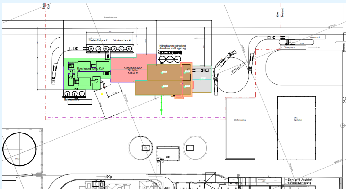
figuur 4: uitbreiding EEW met vierde verbrandingslijn
