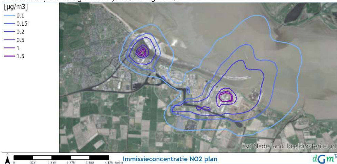
Figuur 25 Immissiecontouren NO 2 voor de toekomstige situatie (plansituatie)
