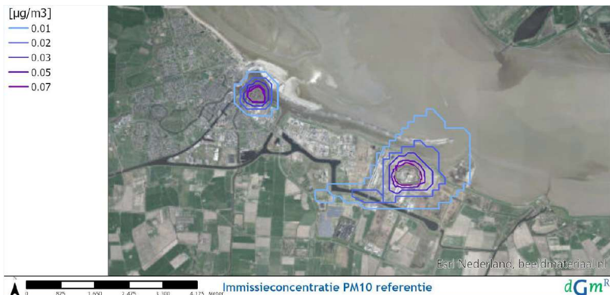
Figuur 24 Immissiecontouren PM 10 voor de referentiesituatie
