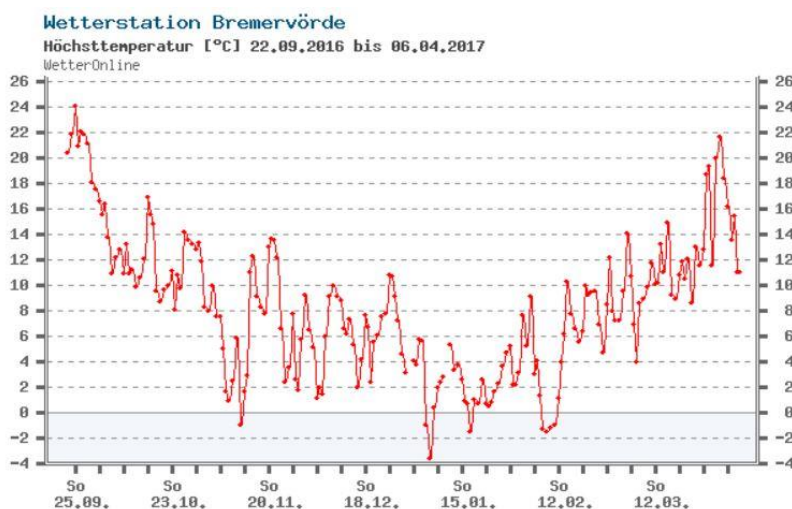
Abbildung 1: Höchsttemperatur in °C in Bremervörde für den Zeitraum 22.09.2016 - 06.04.2017; Quelle: wetteronline.de
