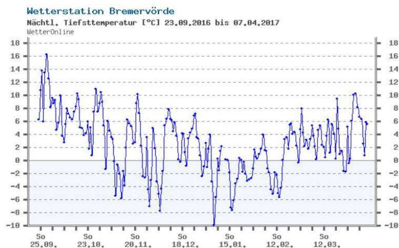
Abbildung 2: Nächtliche Tiefsttemperatur in °C in Bremervörde für den Zeitraum 22.09.2016 - 06.04.2017; Quelle: wetteronline.de
