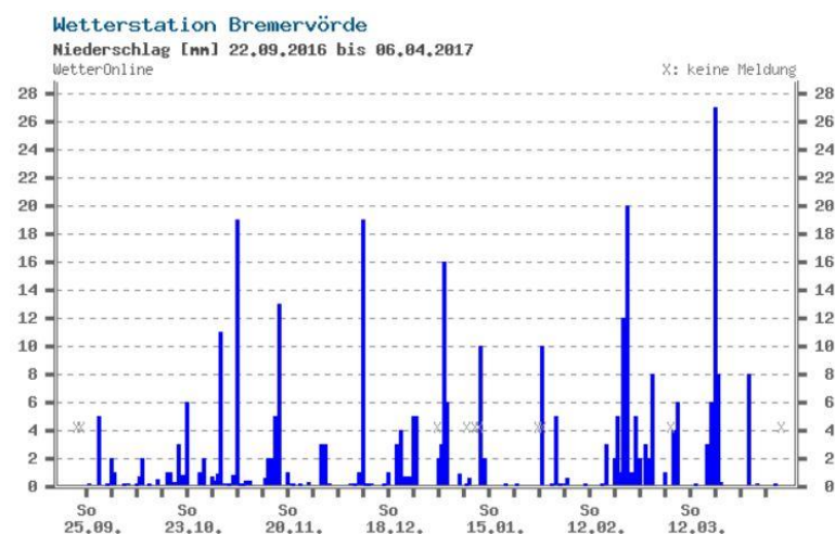
Abbildung 3: Niederschlag in mm in Bremervörde für den Zeitraum 22.09.2016 - 06.04.2017, Quelle: wetteronline.de
