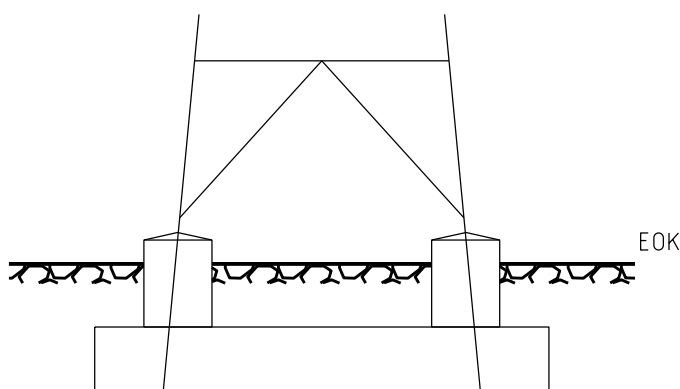
Plattenfundament
