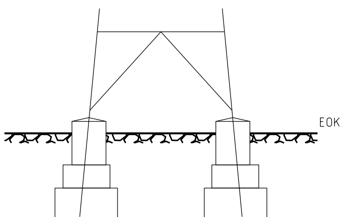
Stufenfundament
