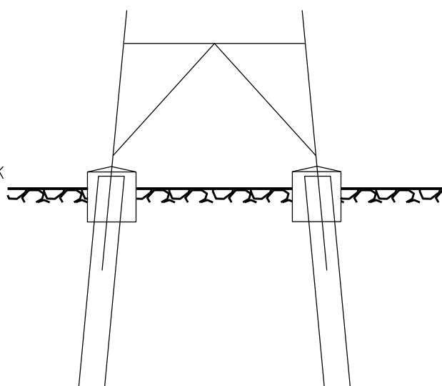
Bohrpfahlfundament
