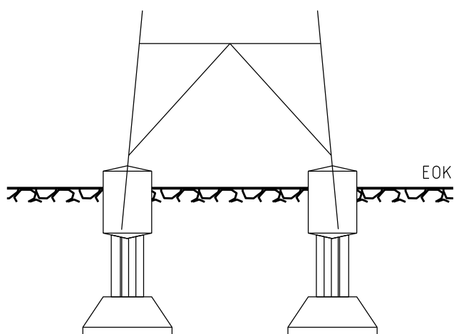
Einsetzfundament
