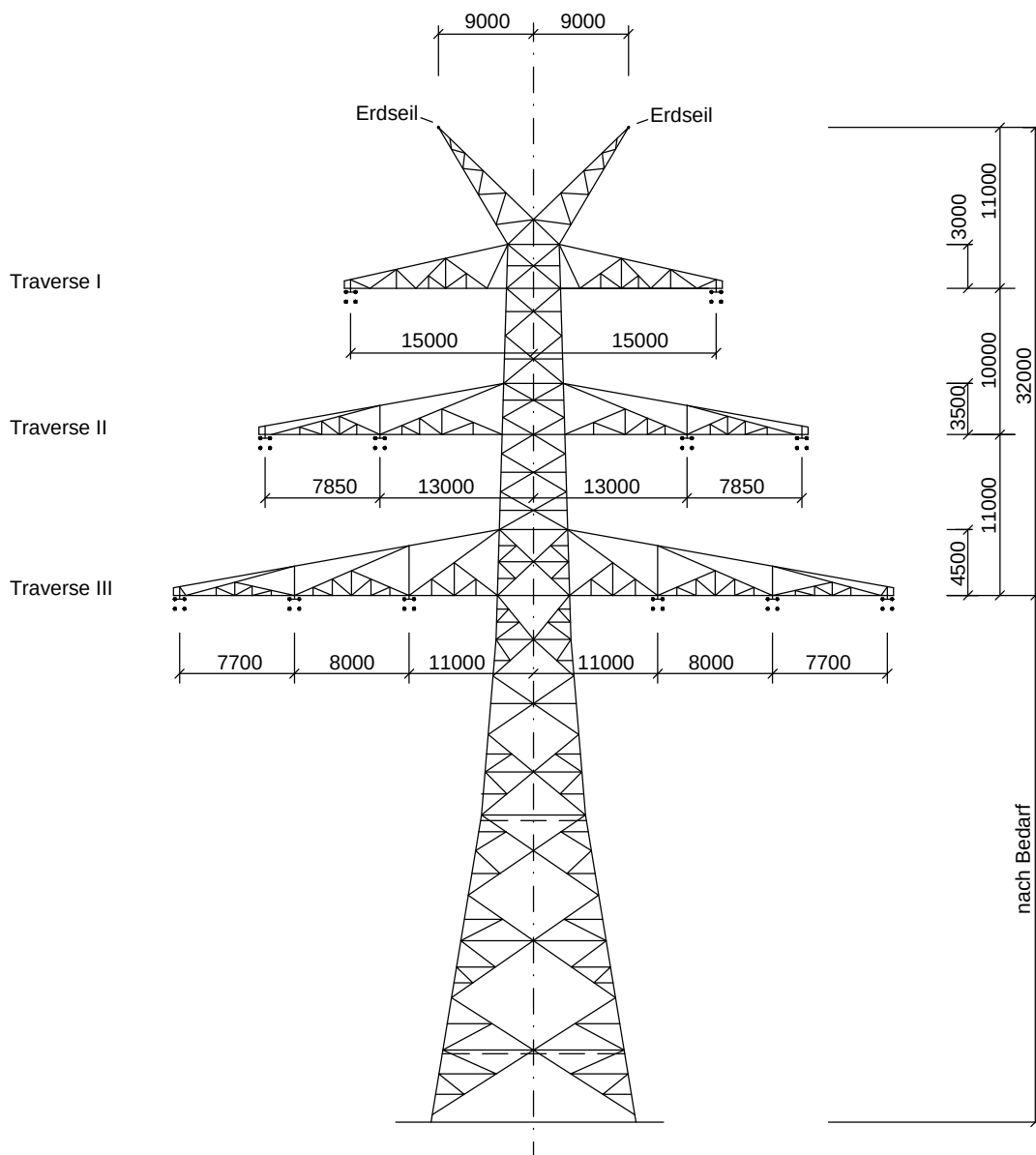
Winkelabspannmast WAspez; DD-4-DE-2008.1 Ltg. Nr. 315: Mast-Nr. 52, 63
