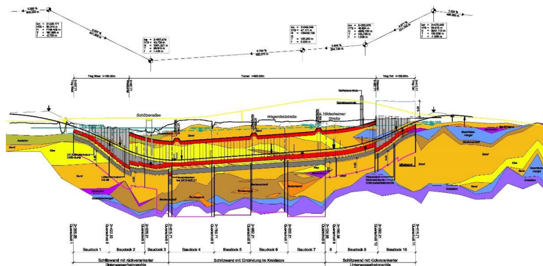
Abbildung 99: Längsschnitt Tunnel und Trog
