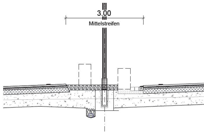
Abbildung 75: Mittelstreifen mit Lärmschutzwand zwischen dem Ostportal und dem Bestandstrog
