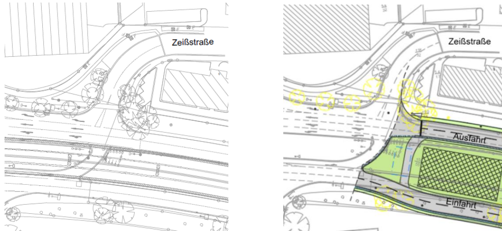
Abbildung 65: Knotenpunkt stlich Hildesheimer Strae / Zeistrae. Links Bestand, rechts Wiederherstellung
