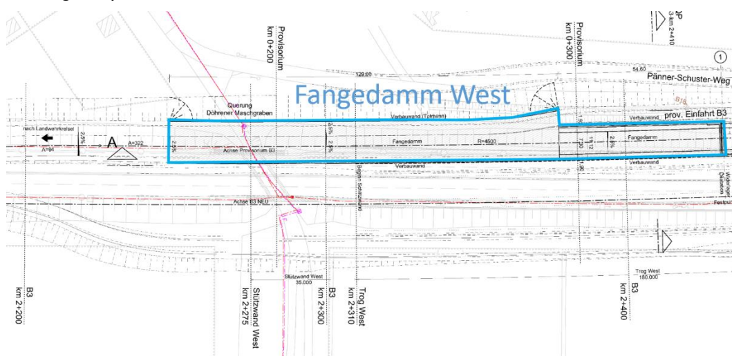
Abbildung 109: Fangedamm West
