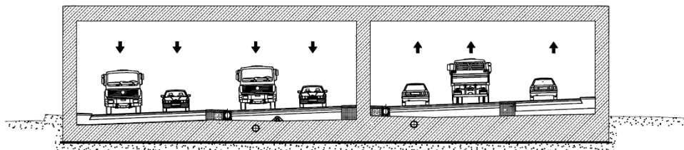
Abbildung 31: Ein- und Ausfahrten im Bereich der Einhausung (Gradiente O3A) ca. Bau-km 3+600
