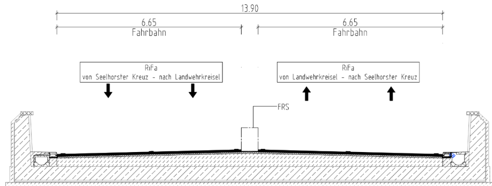
Abbildung 117: Querschnitt des Trops unter den DB-Brücken nach dem Umbau auf das Dachprofil
