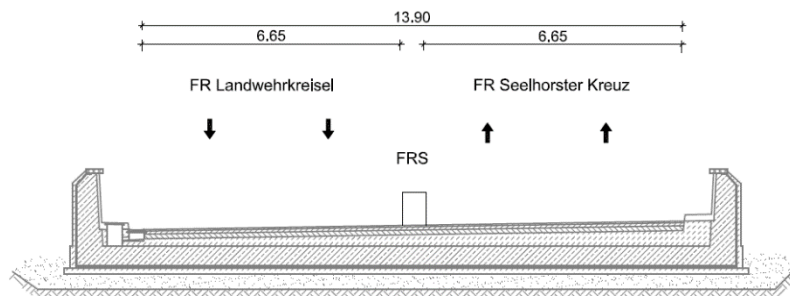
Abbildung 70: Bestandstrog unter den DB-Brücken mit vorhandener Einseitneigung
