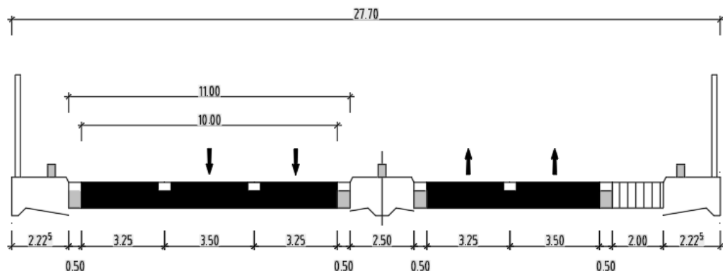
Abbildung 112: Querschnitt Geh- und Radwegunterführung Mühlenholzweg
