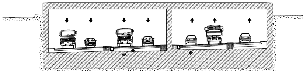
Abbildung 32: Ein- und Ausfahrten im Bereich der Einhausung (Gradiente O3B) ca. Bau-km 3+600 (Verstärkte Sohlplatte zur Sicherung gegen Auftrieb)
