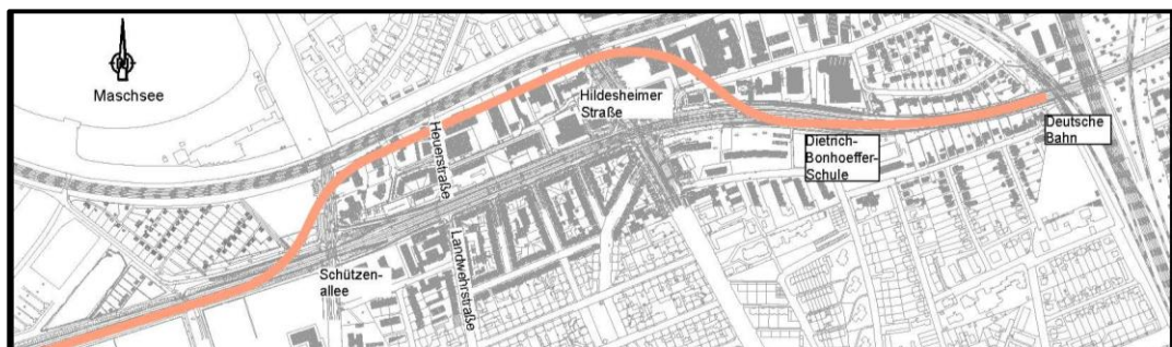
Abbildung 16: Variante O2 „Dammlage nördlich abgerückt“
