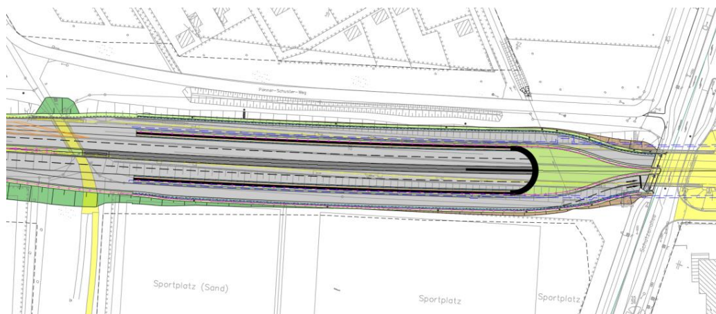
Abbildung 85: Geplante Ein- und Ausfahrrampen westlich der Schützenallee
