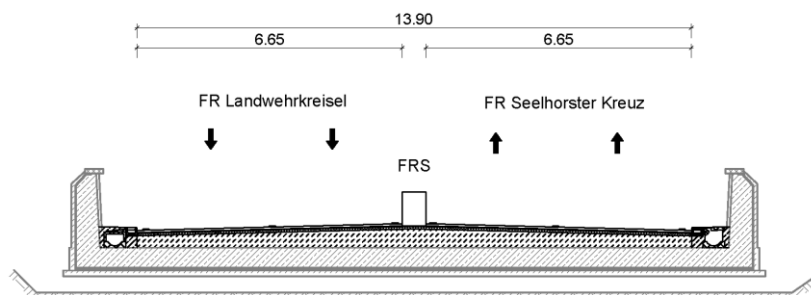
Abbildung 71: Bestandstrog unter den DB-Brücken umgebaut auf Dachprofil
