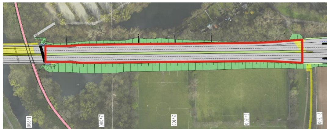
Abbildung 134: Entwässerungsabschnitt 7
