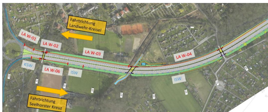
Abbildung 118: Übersicht Lärmschutzanlagen und Irritationsschutzwände im West-Bereich (Landwehrkreisel bis Unterführung Bauernwiese)
