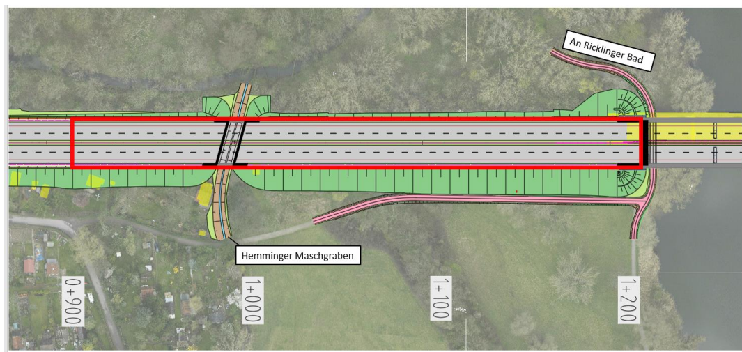
Abbildung 130: Entwässerungsabschnitt 3
