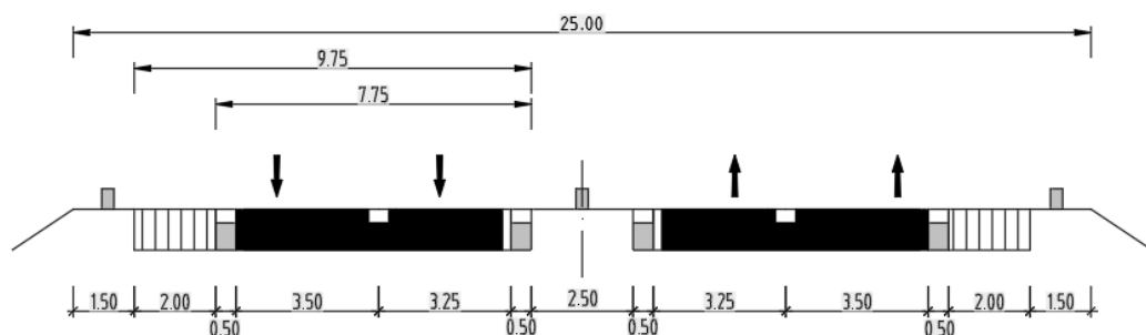
Abbildung 56: Regelquerschnitt RQ 25
