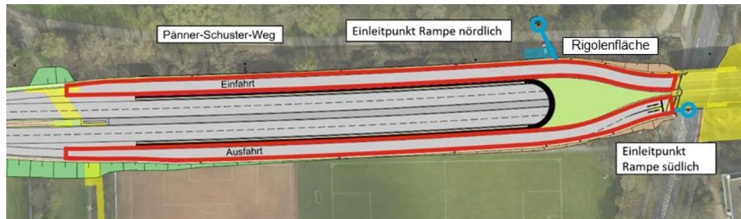
Abbildung 135: Entwässerungsabschnitt 8
