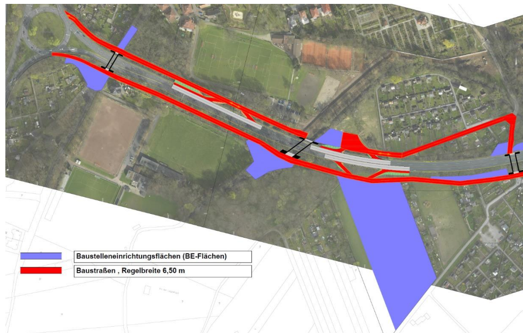
Abbildung 151: Vorgesehene Baustraßen und BE-Flächen im Bereich zwischen Landwehrkreisel und der Brücke „An der Bauerwiese“ (BW 03)
