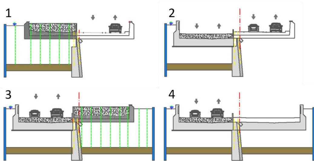
Abbildung 116: Prinzipieller Bauablauf der Verbreiterung des Bestandstrogs unter Verkehr
