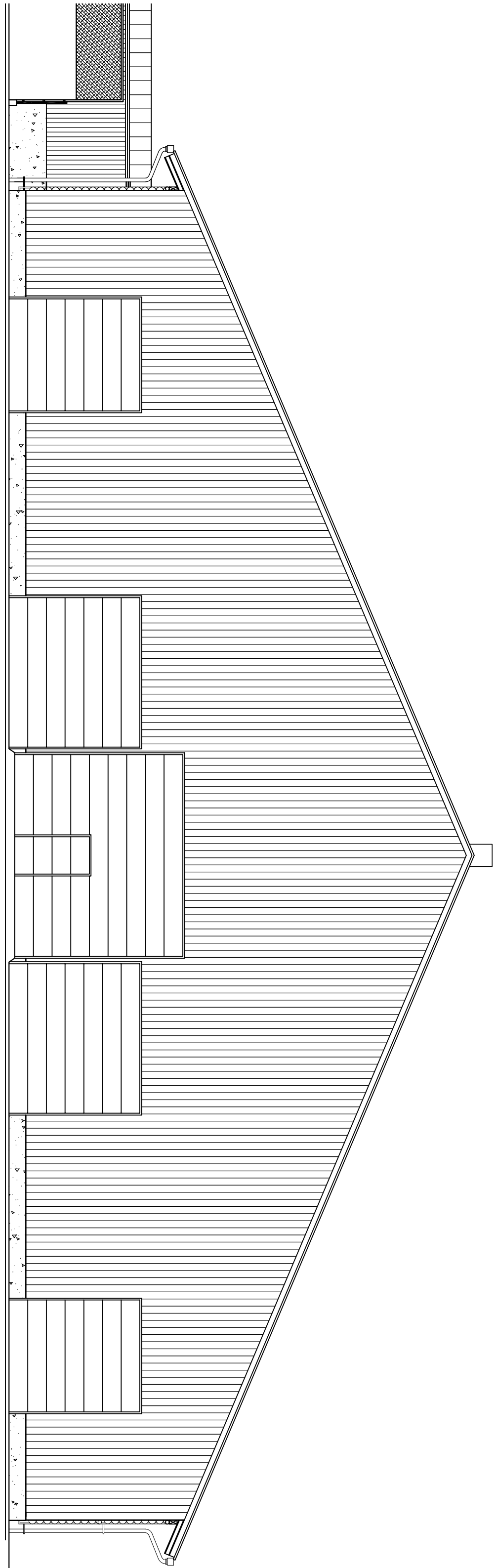
Südansicht
