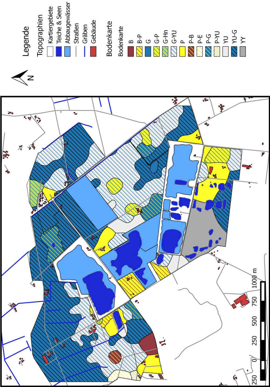
Abb. 3: Bodentypenkarte
