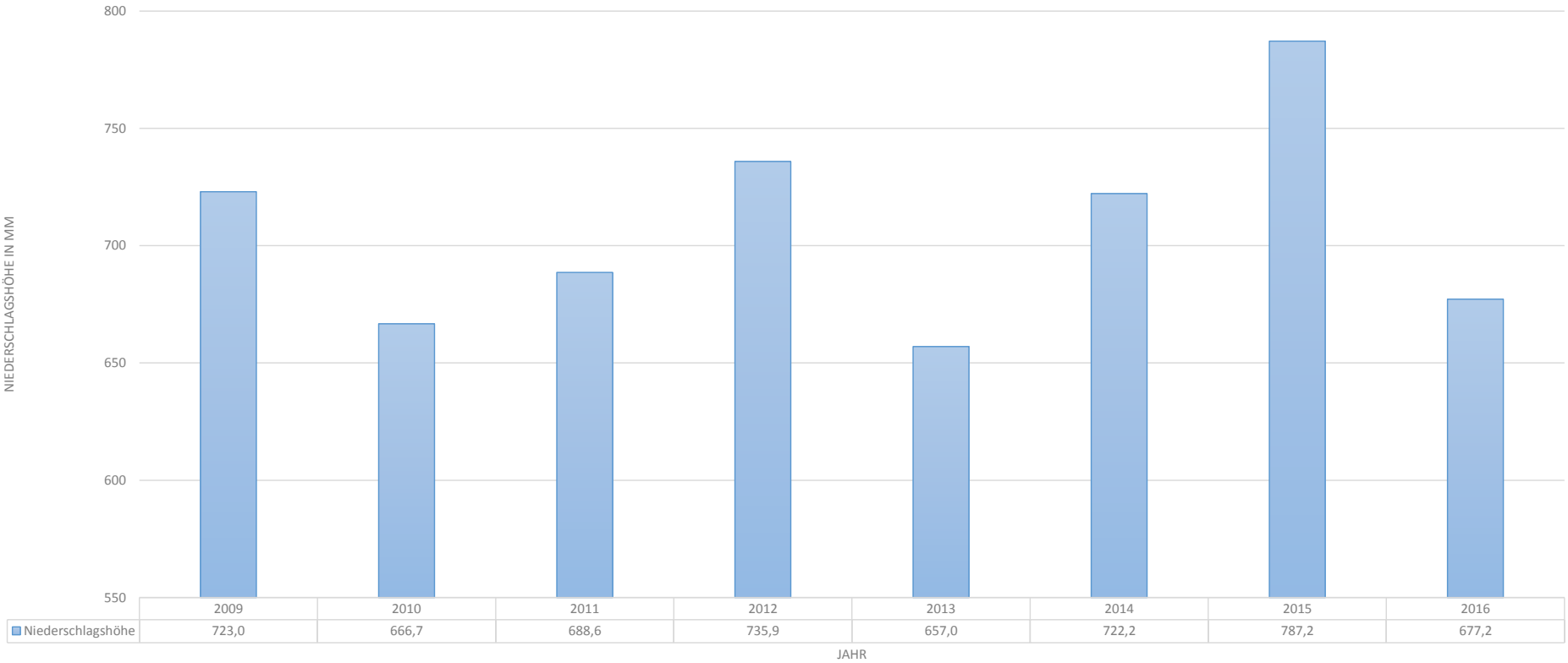
Niederschlag 2009 - 2016, Station Lingen
