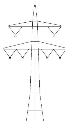
Tragmast Donau mit Erd- seilspitze D-2-D-2015.3 2018.3
