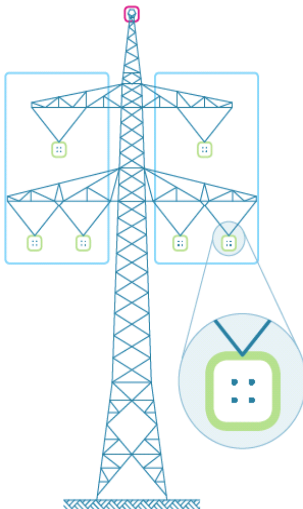
Abbildung 10: Beseilung am Freileitungsmast
