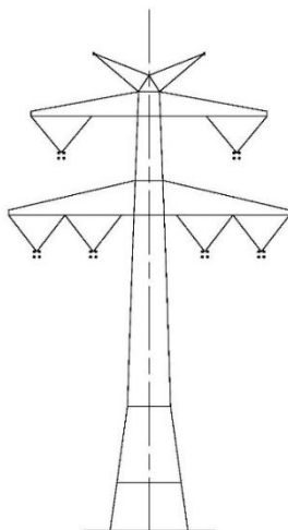
Tragmast Donau mit Erd- seilhörn geteilter ES D-2-D-2015.3 2018.3
