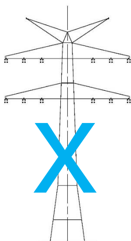
Abspannmast Einebene- kreuztraverse Traverse 2 90° gedreht Erdseilhörn D-2-E-2016.1
