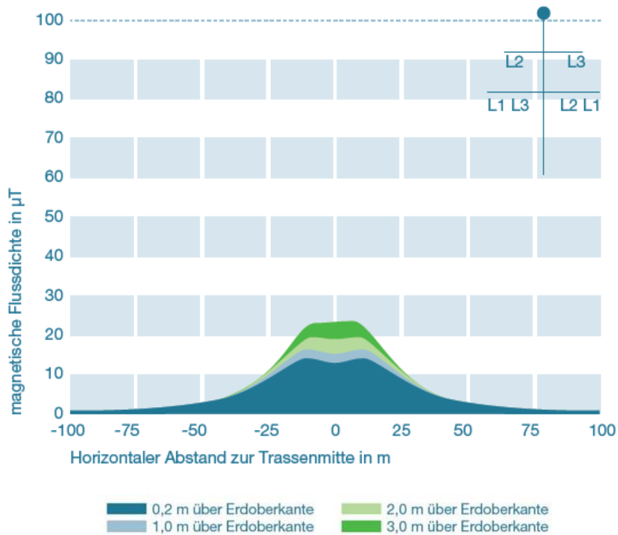
Abbildung 14: Magnetische Felder bei der Freileitung
