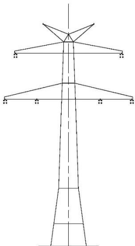
Abspannmast Donau mit Erdseilhörn geteilter ES D-2-D-2015.3 2018.3
