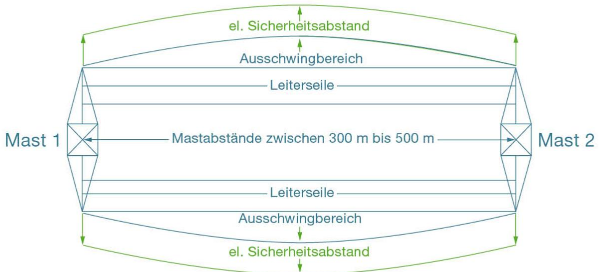
Abbildung 13: Schutzstreifen (schematische Darstellung in der Draufsicht)
