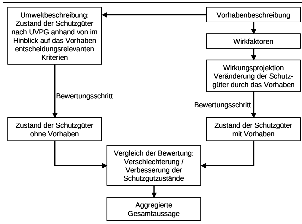
Abb. 1: Vorhaben-Umwelt-Modell - Vorgehensweise
