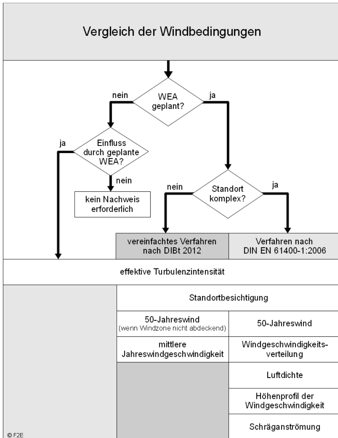
Abbildung 2.1.1: Nachweis durch Vergleich der Windbedingungen gemäß /17/.
