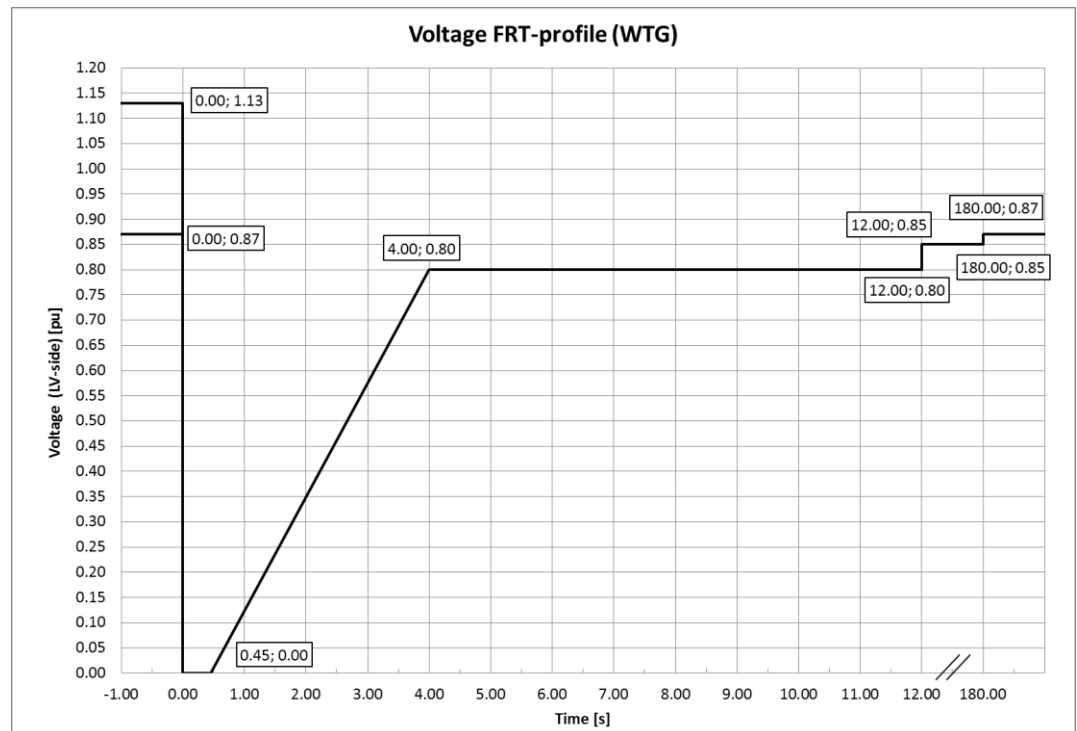
Abbildung 10-2: Niedrige Spannungstoleranzkurve für symmetrische und asymmetrische Störungen, wobei U die gemessene Spannung im Stromnetz darstellt.
