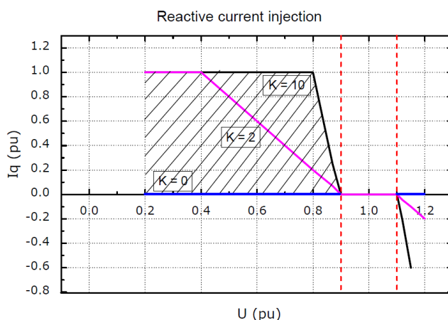
Abbildung 10-3: Blindstromeinspeisung
