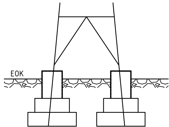
Stufenfundament
