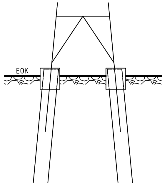
Rammpfahlgründung
