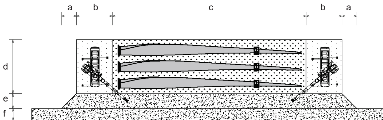
Abb. 10: Rotorblattlagerfläche (Konstruktionsschema)
