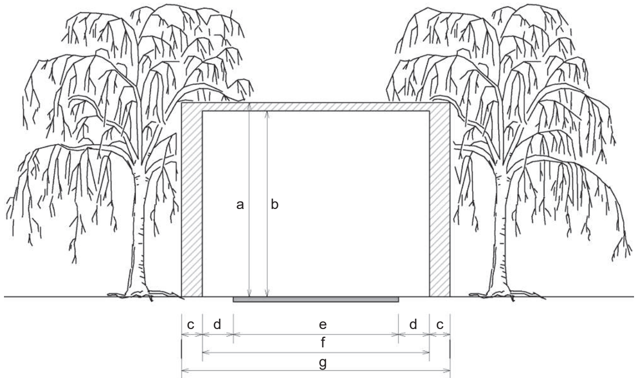
Abb. 5: Lichtraumprofil
