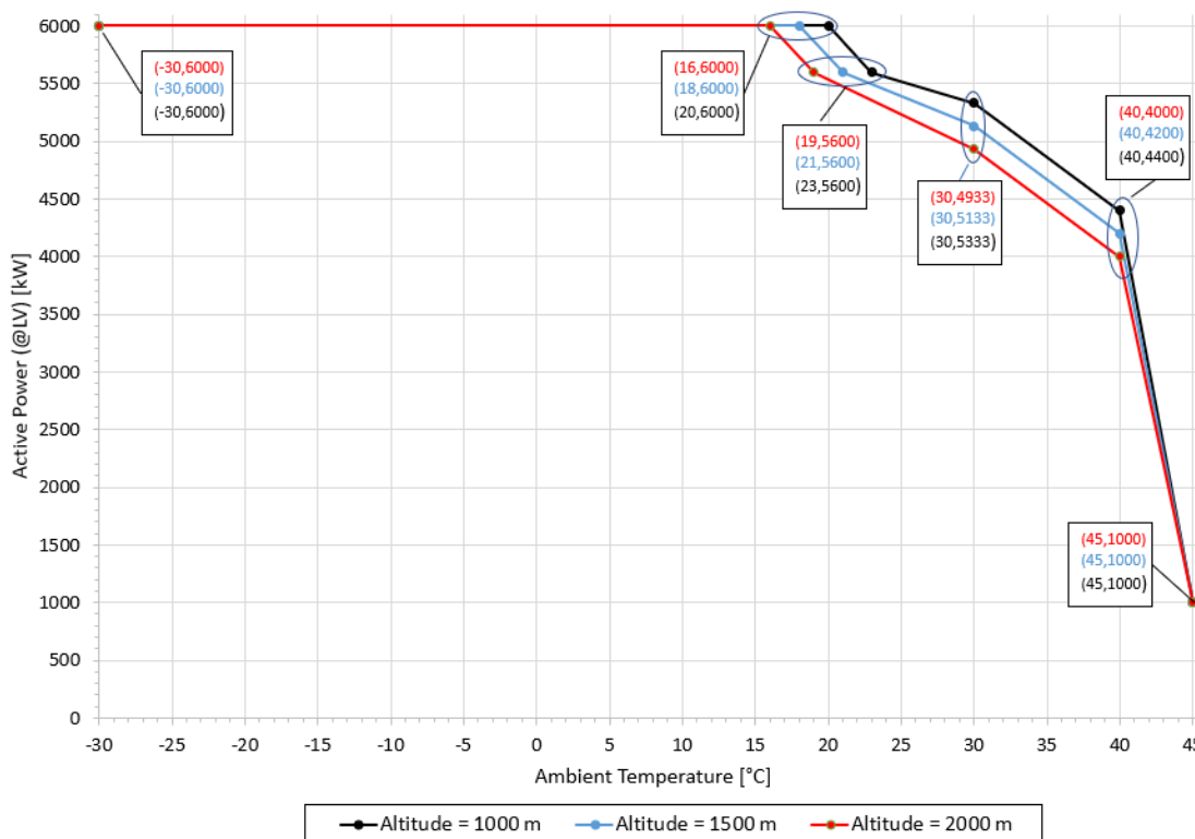
Abbildung 3-1: Temperaturabhängiger gedrosselter Betrieb
