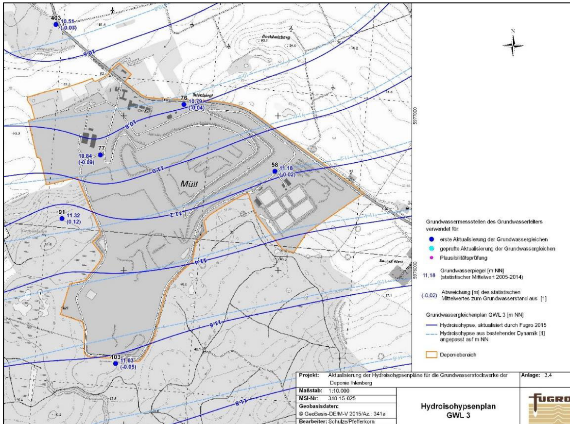
Abbildung 4: Grundwassergleichenplan GWL 3 (statistische Mittelwerte 2005 - 2015) [3]
