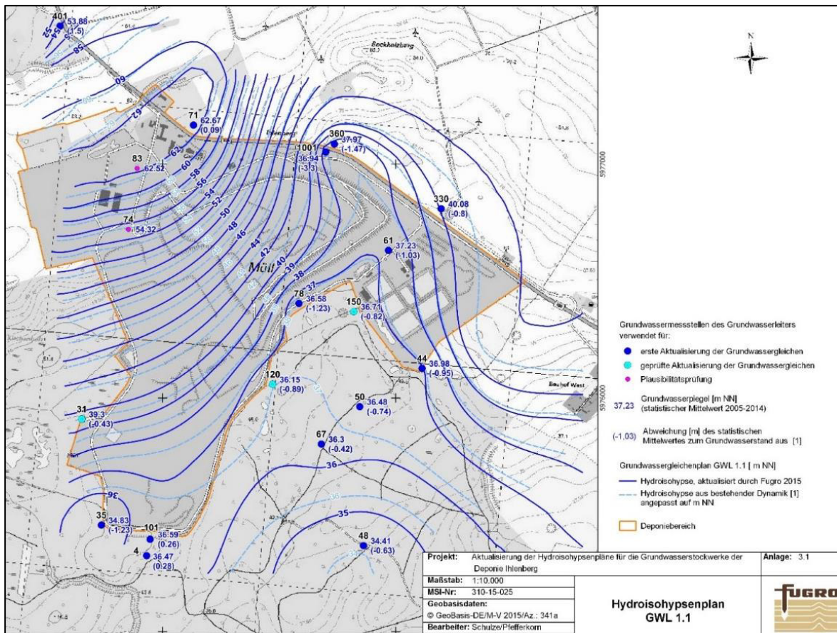
Abbildung 1: Grundwassergleichenplan GWL 1.1 (statistische Mittelwerte 2005 - 2015) [3]
