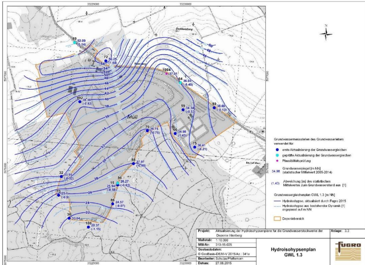
Abbildung 3: Grundwassergleichenplan GWL 1.3 (statistische Mittelwerte 2005 - 2015) [3]
