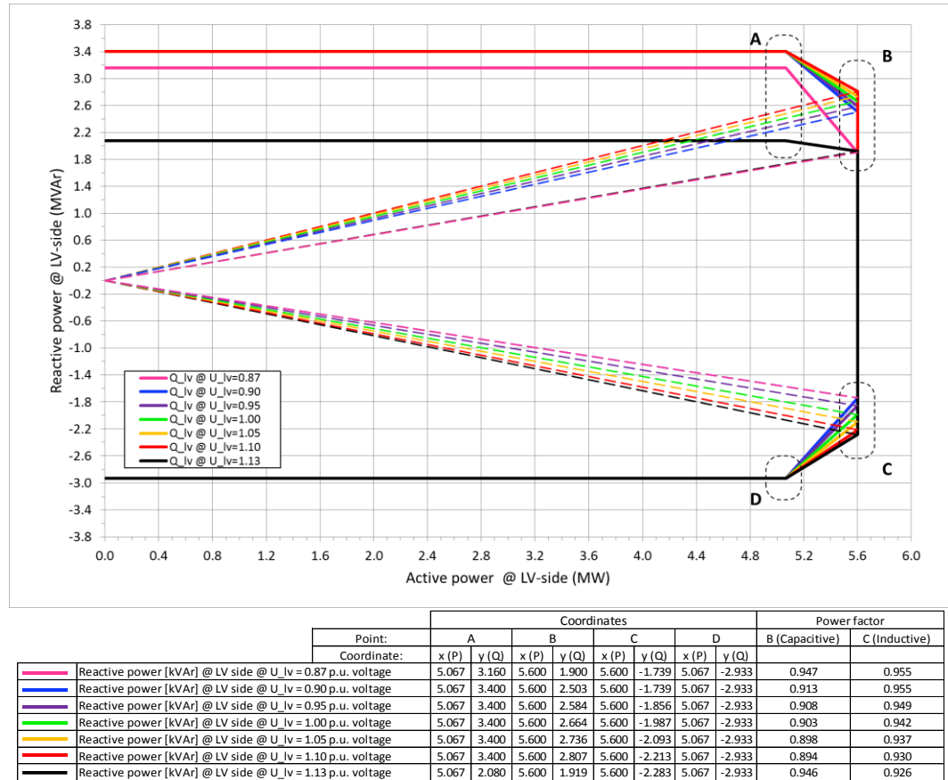
Abbildung 3-2: Blindleistungskapazität.
