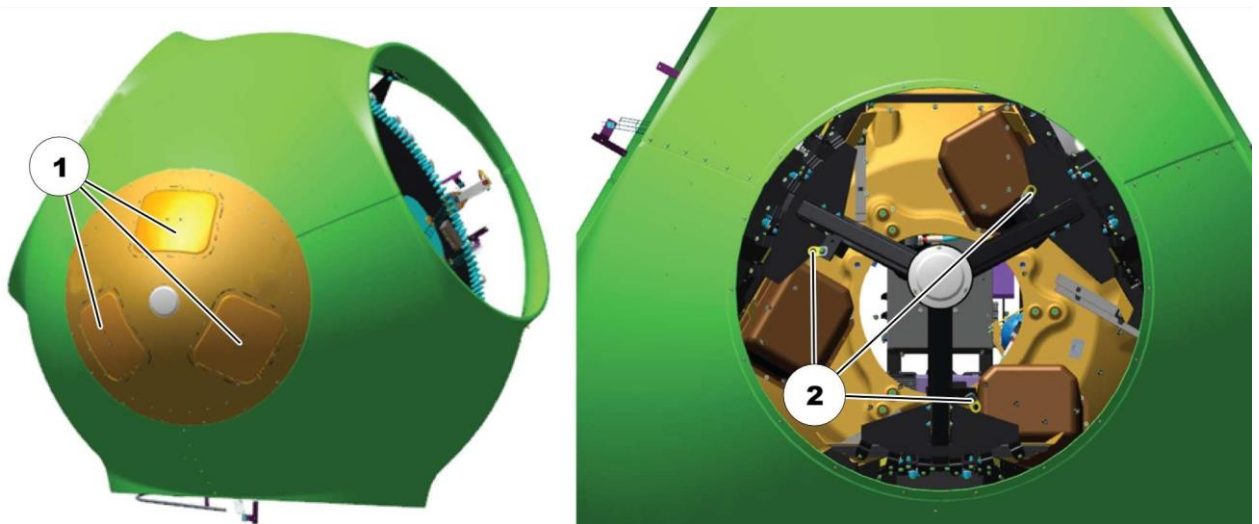
Abbildung 5.19: Rettungsweg durch die Spinnerluken und die Anschlagpunkte für die Abstiegsvorrichtung
