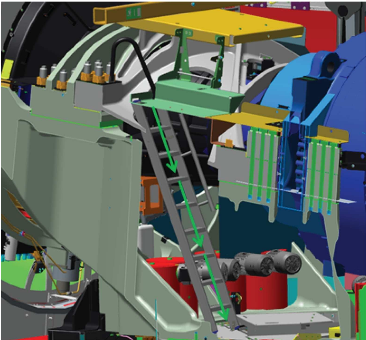
Abbildung 5.7: Evakuierungsroute vom Maschinenhaus über die Leiter zum Azimutdeck
