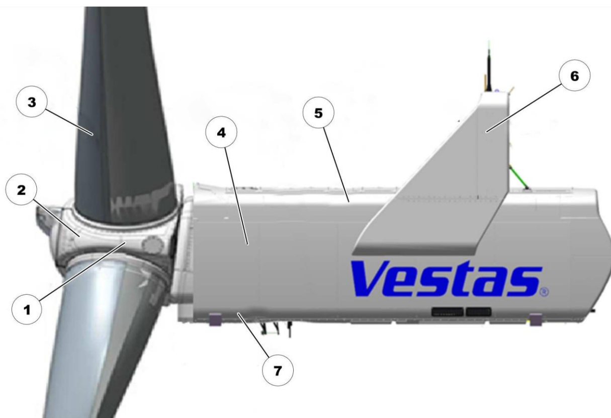
Abbildung 5.2: Maschinenhausbereiche
