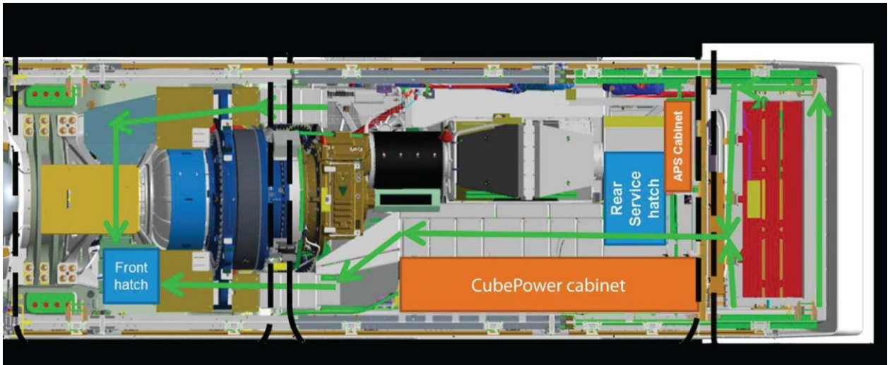
Abbildung 5.6: Evakuierungsroute im Maschinenhaus
