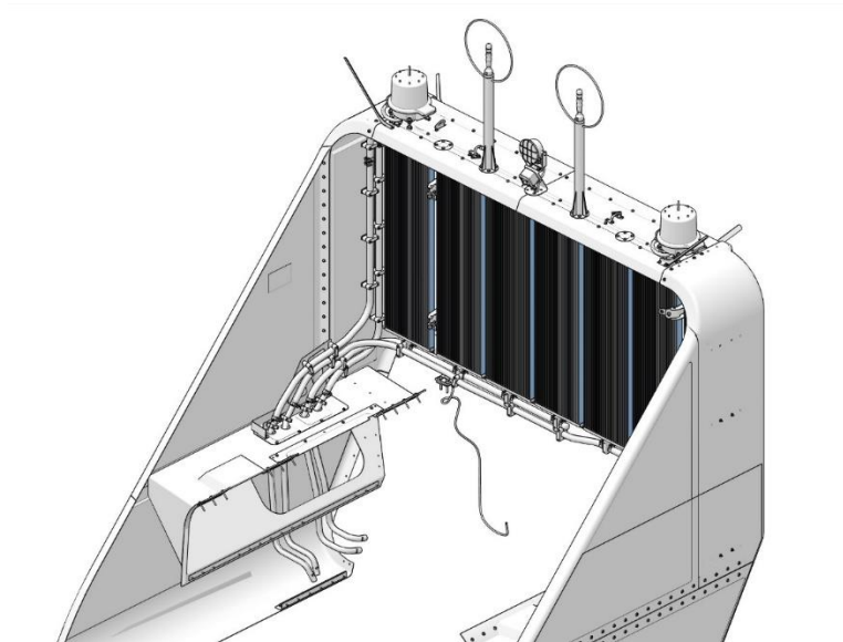
Abbildung 3-3 Darstellung von Ultraschall-Anemometer und Gefahrenfeuer am CoolerTop® an der Rückseite des Maschinenhausdaches beschrieben.
