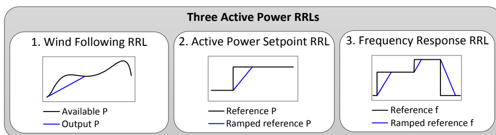
Abbildung 4-7: Drei Wirkleistungs-RRL
