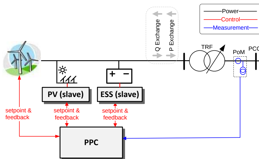
Abbildung 4-4: Option 4 Regelarchitektur mit WEA, PV und/oder ESS
