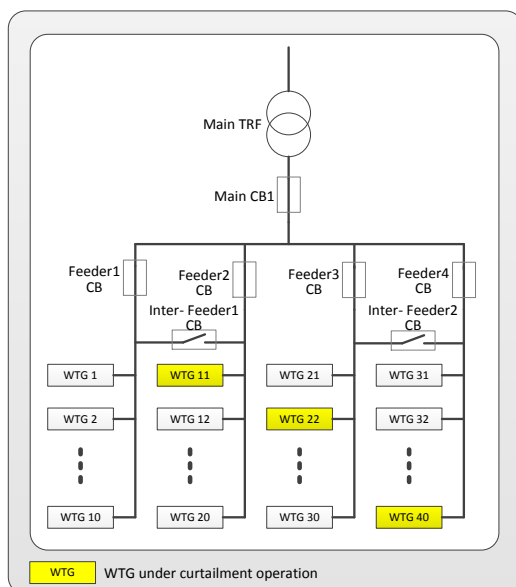
Abbildung 4-9: Beispiel für den Gruppen-Leistungsgrenzwert
