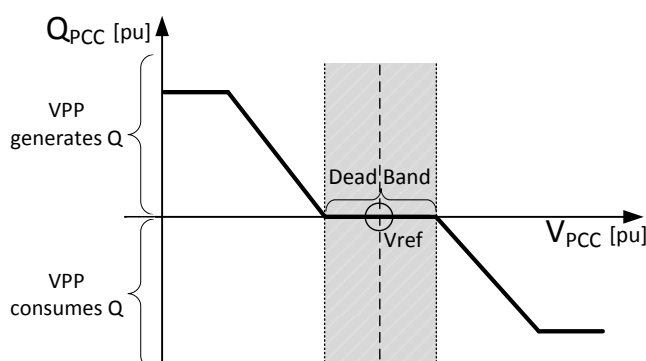
Abbildung 4-6: Merkmale des Spannungsreglers
