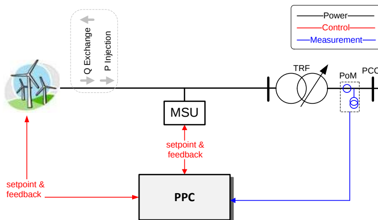
Abbildung 4-2: Option 2: Regelarchitektur mit WEA und MSU
