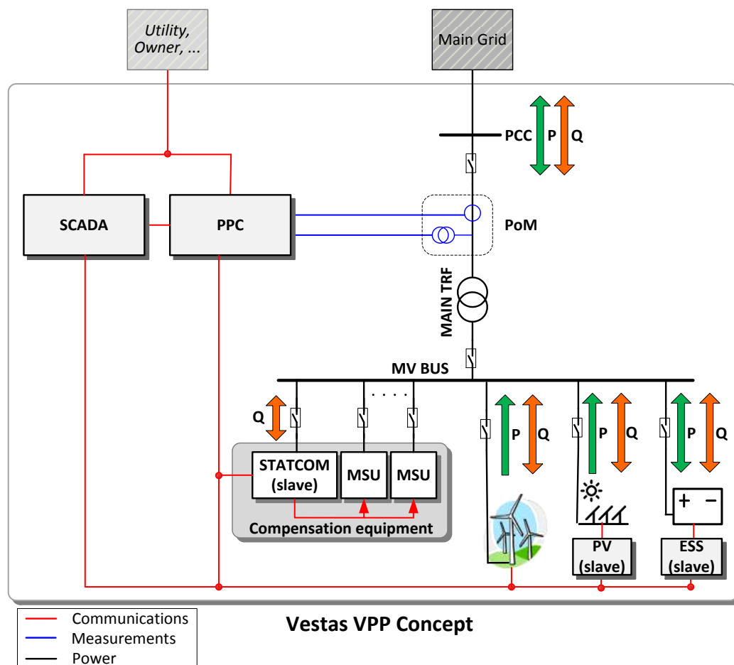
Abbildung 3-1: Beispiel für eine Vestas Windpark-Architektur mit VestasOnline®-PPC
