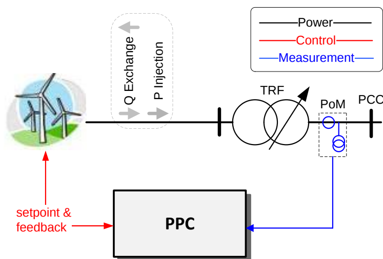
Abbildung 4-1: Option 1: Regelarchitektur lediglich mit WEA
