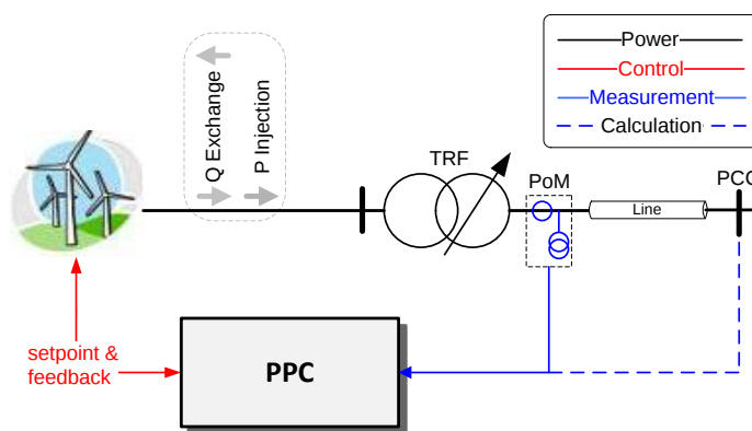
Abbildung 4-10: Kompensationssteuerung bei Spannungsabfall für Vestas-Option 1
