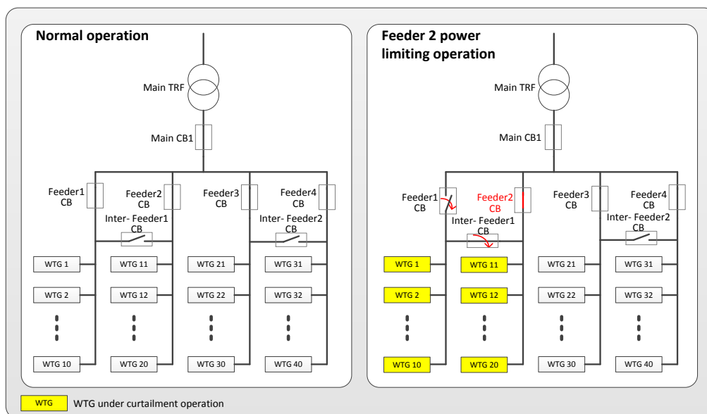
Abbildung 4-8: Beispiel für die Funktionsweise eines PPC zur Begrenzung des Einspeisestroms
