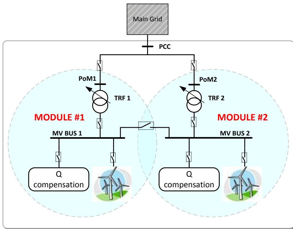
Abbildung 4-5: Beispiel für einen aus zwei gleichartigen Modulen aufgebauten Vestas-Windpark
