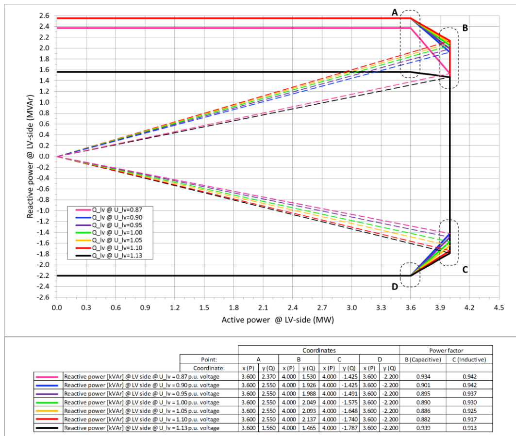
Abbildung 10-2: Blindleistungskapazität im 4,0-MW-Modus 0.
