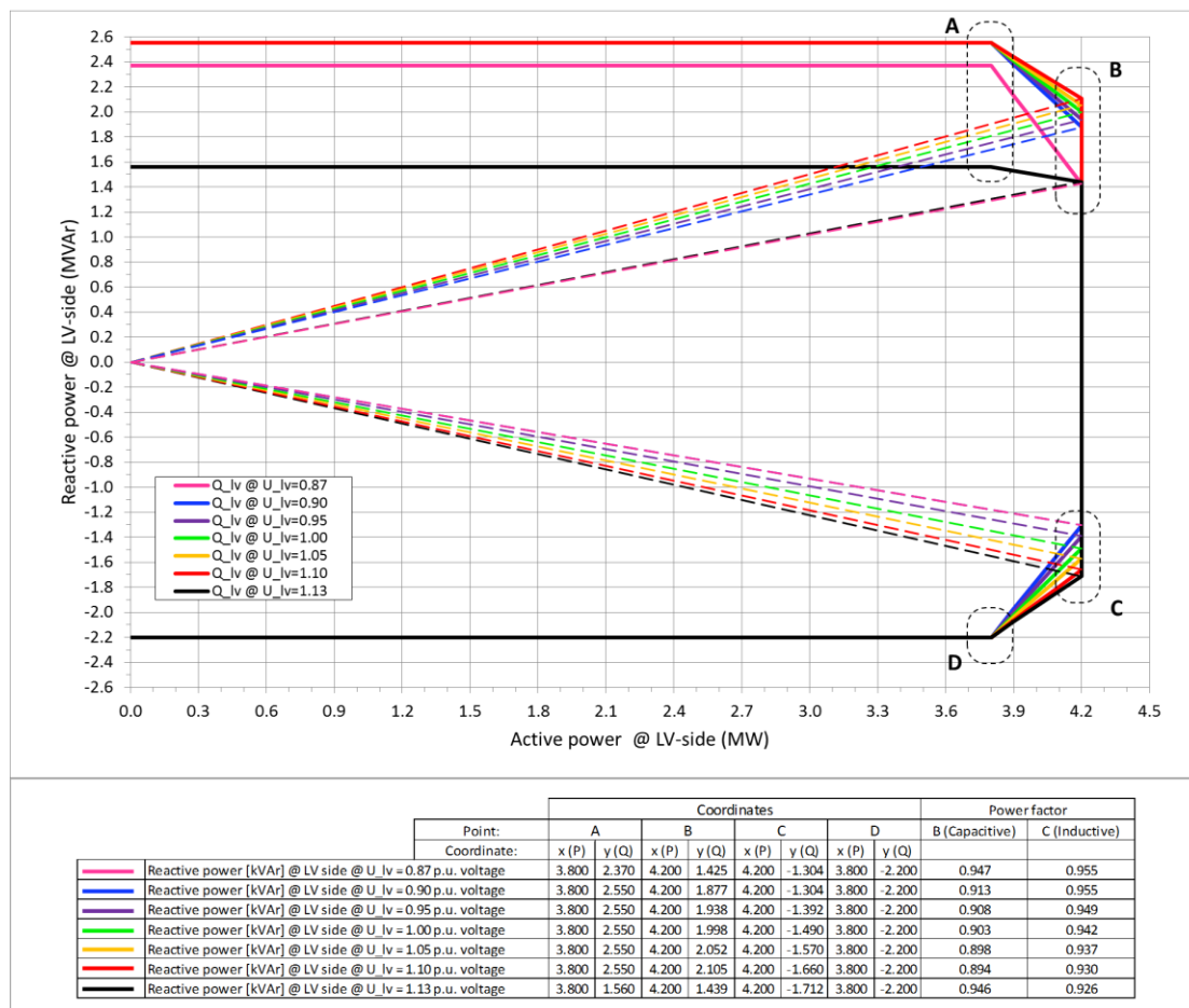
Abbildung 10-4: Die Blindleistungskapazität im leistungsoptimierten 4,2-MW-Modus (PO1).
