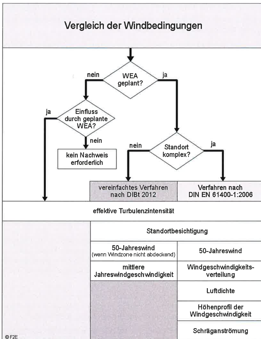
Abbildung 2.1.3: Nachweis durch Vergleich der Windbedingungen gemäß /2.8/.
