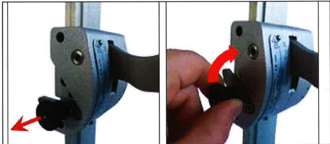
Abb. 12: Fallschutzläufer Sperre
