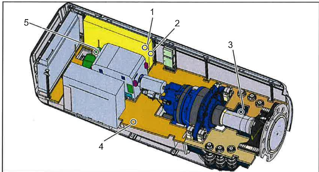
Abb. 15: Not-Halt-Schalter und Ausschalter Mittelspannung im Maschinenhaus
