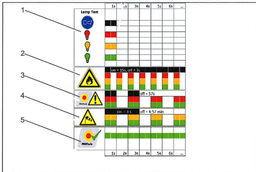
Abb. 18: Bedeutung der Signalmuster
