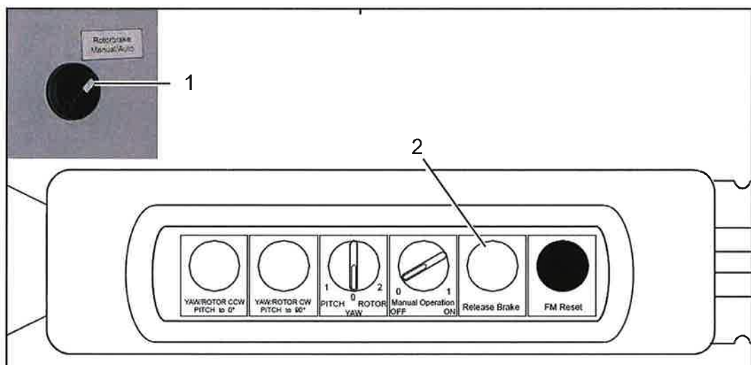
Abb. 22: Bedienelemente für manuellen Betrieb der Rotorbremse
