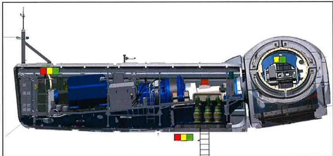
Abb. 17: Position der Signalleuchten
