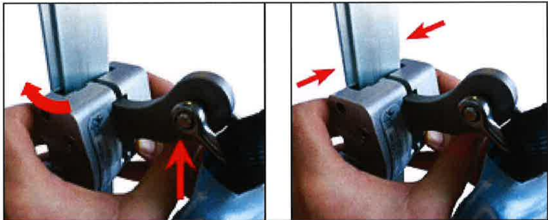
Abb. 11: Fallschutzläufer an die Fallschutzschiene angelegt
