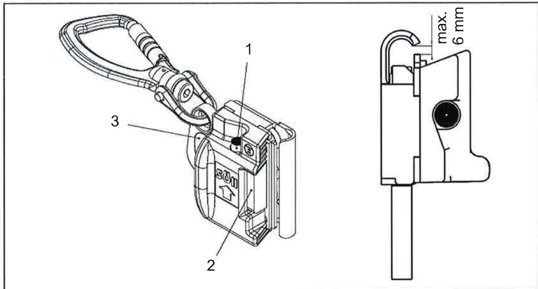
Abb. 13: Fallschutzläufer des Vi-Go-Systems
