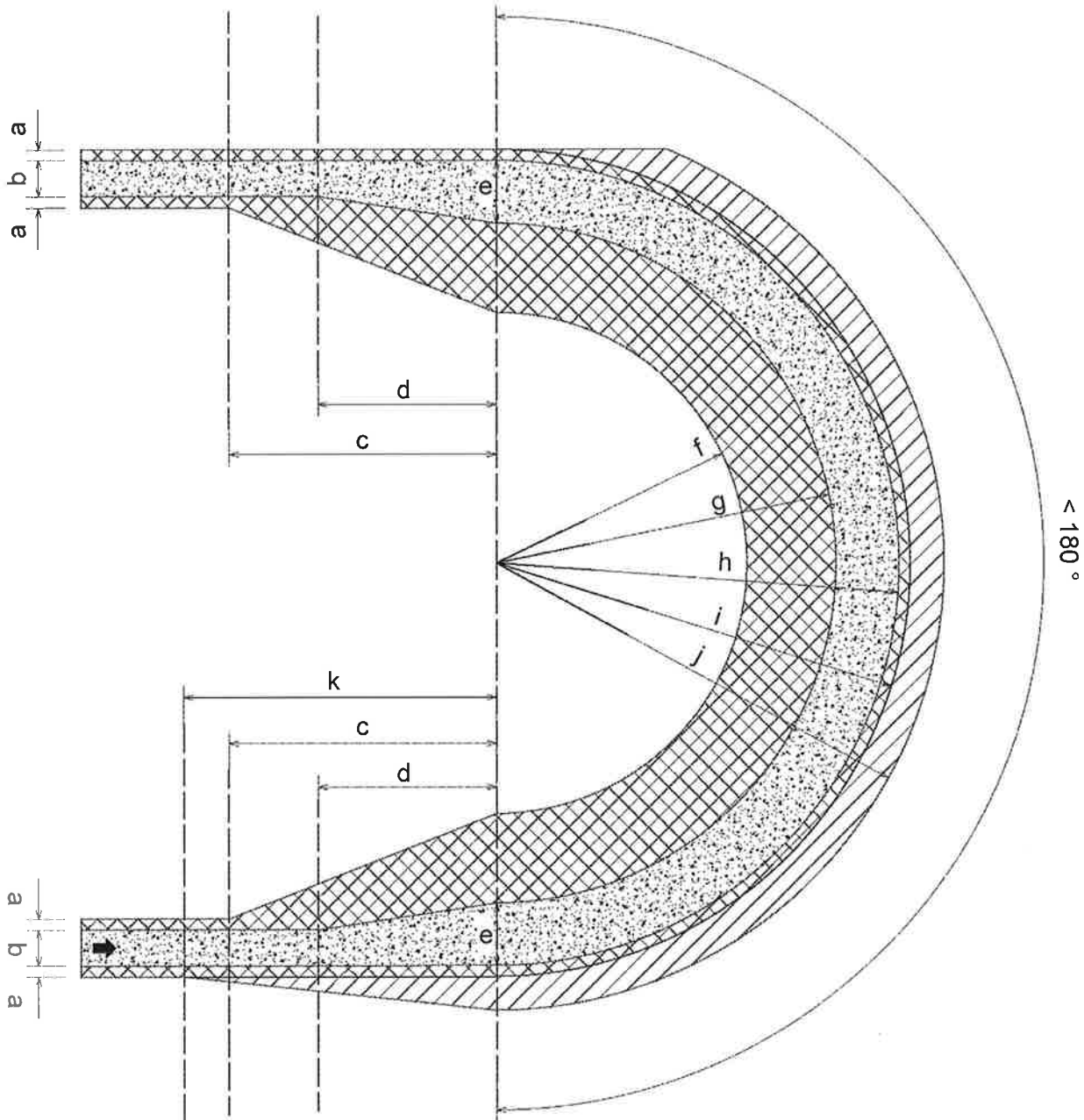
Abb. 3: 180-Grad-Kurve (Konstruktionsschema)
