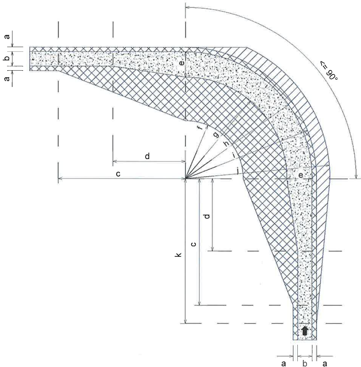
Abb. 2: 90-Grad-Kurve (Konstruktionsschema)
