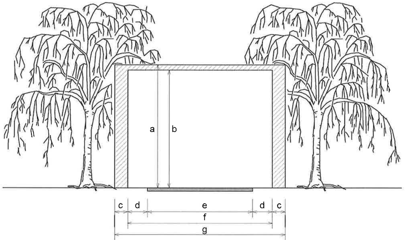
Abb. 5: Lichtraumprofil
