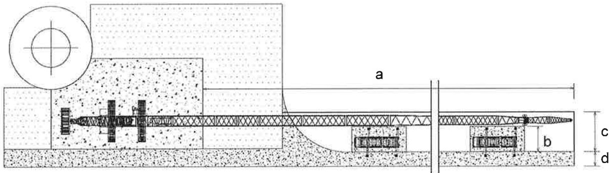
Abb. 9: Kranauslegermontagefläche
