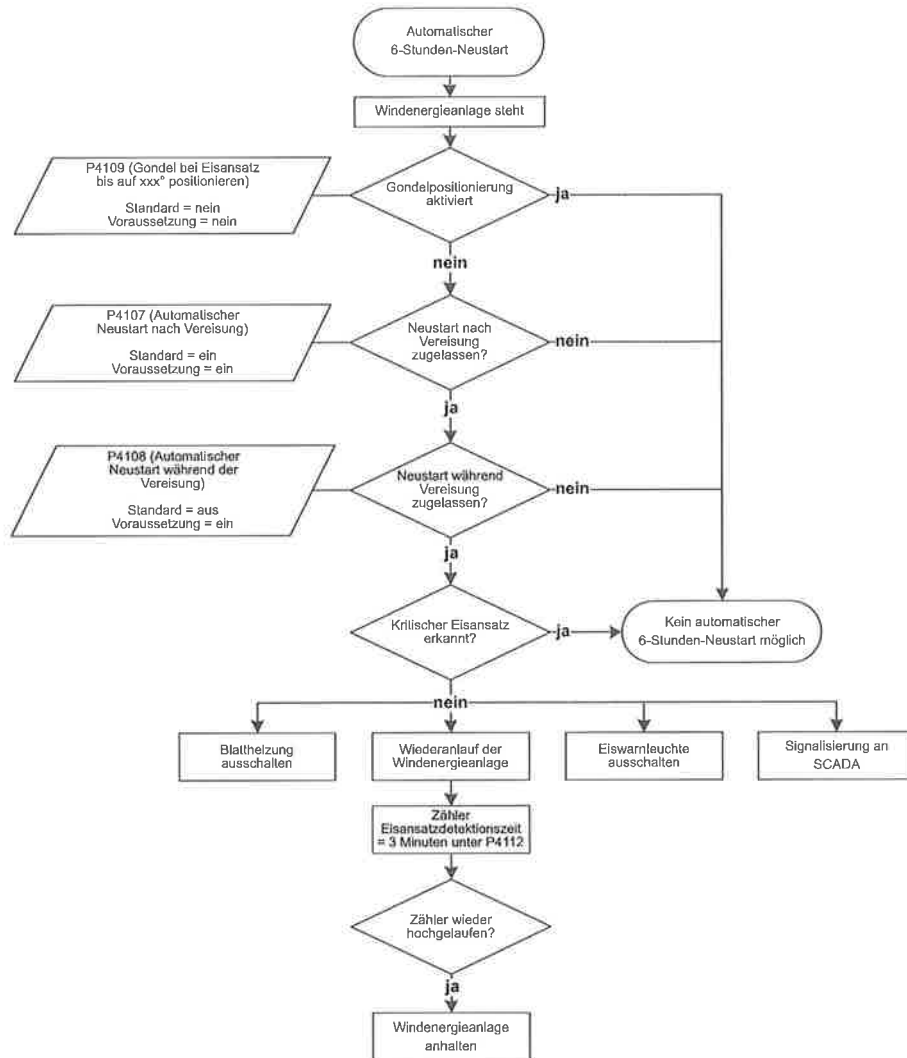
Abb. 2: Automatischer 6-Stunden-Neustart
