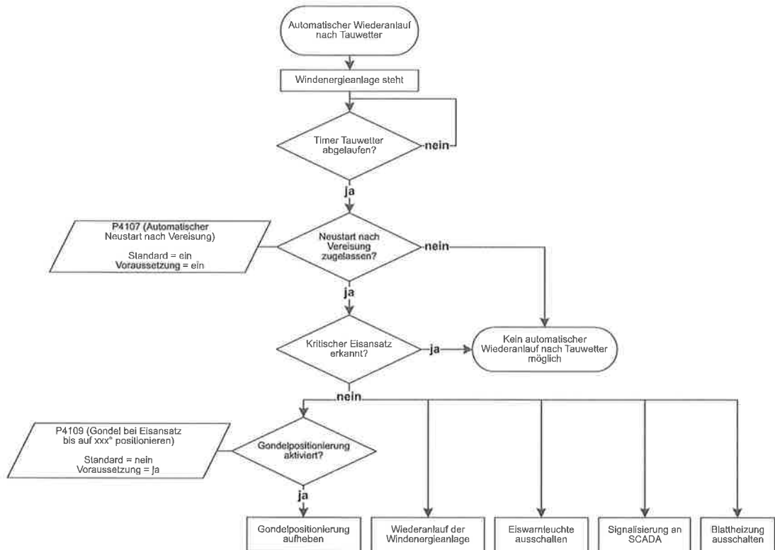
Abb. 1: Automatischer Wiederanlauf nach Tauwetter
