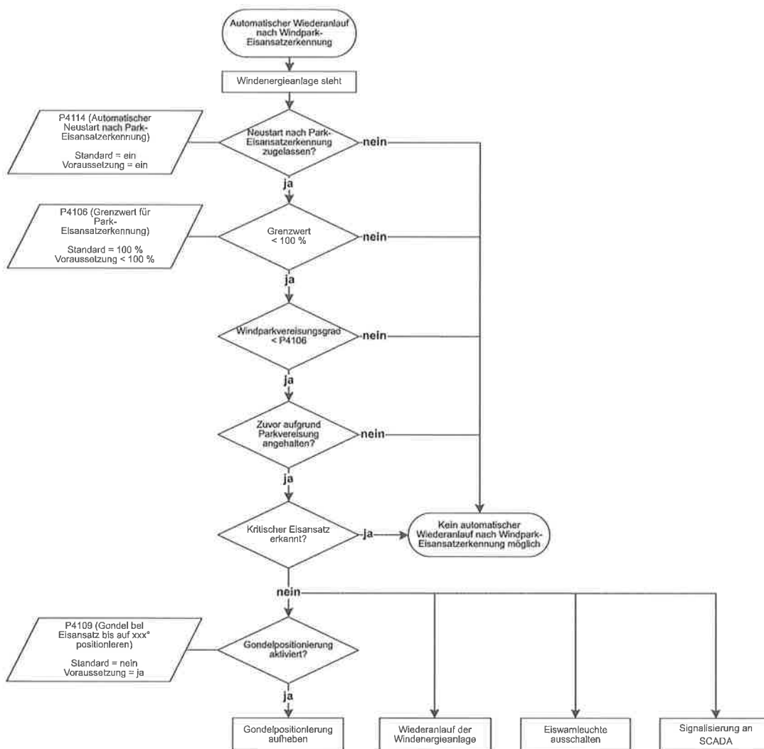
Abb. 4: Automatischer Wiederanlauf nach Windpark-Eisansatzerkennung
