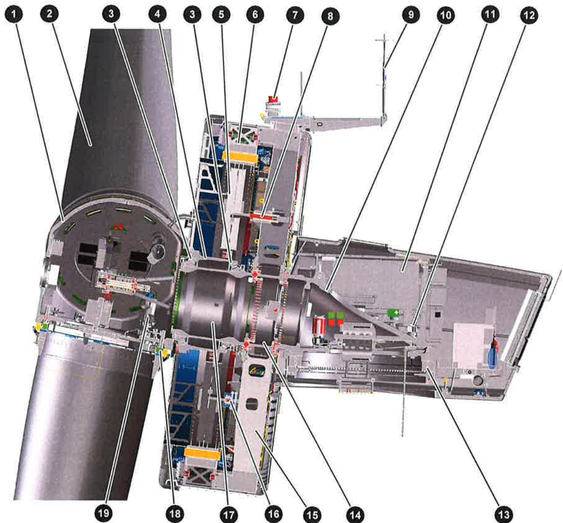
Abb. 2: Gondelschnitt
