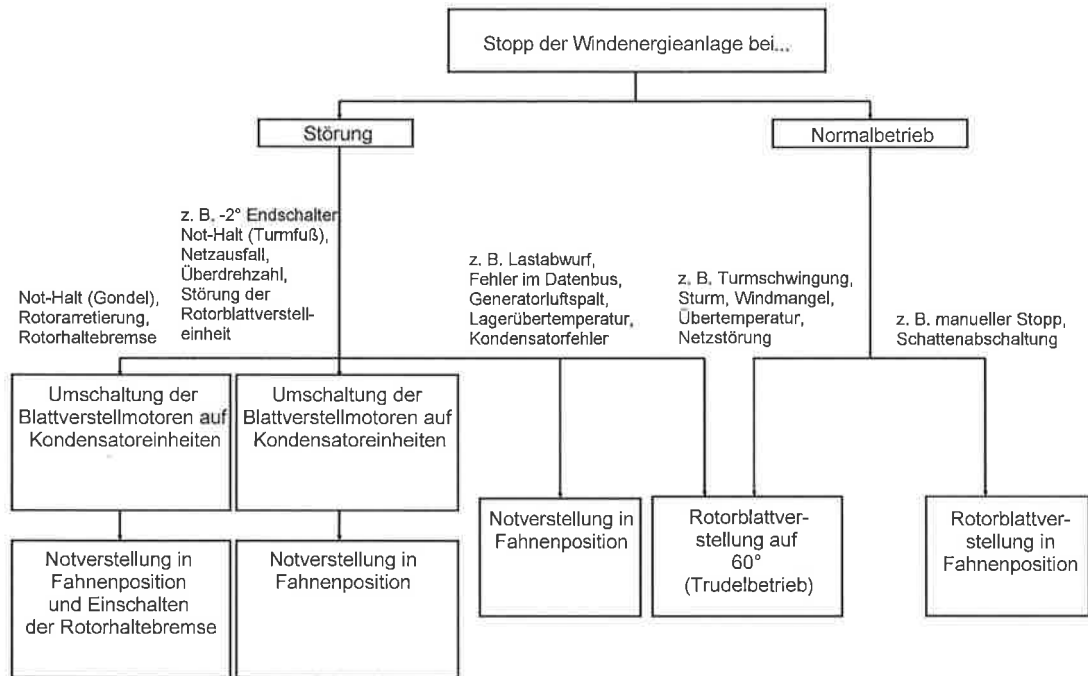
Abb. 5: Übersicht Windenergieanlagenstopp
