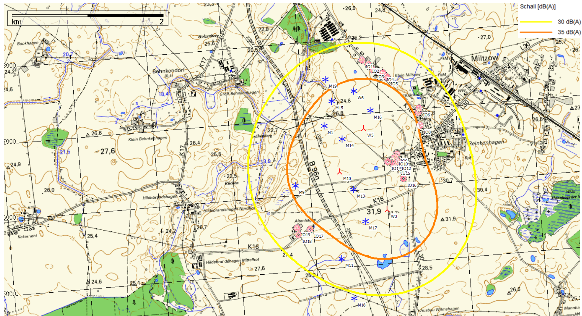
Abbildung 9.1: Einwirkungsbereich der geplanten WEA Vestas V112-3.3/3.45MW Mode 8+ Schall – Isolinie (nachts)
