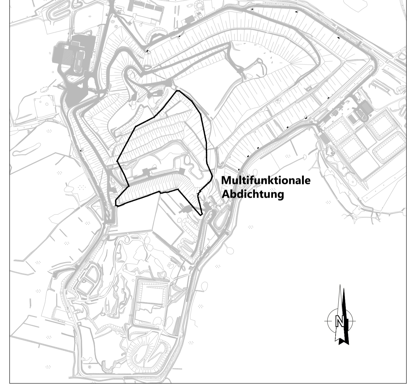
Übersichtslageplan M 1 : 10.000
