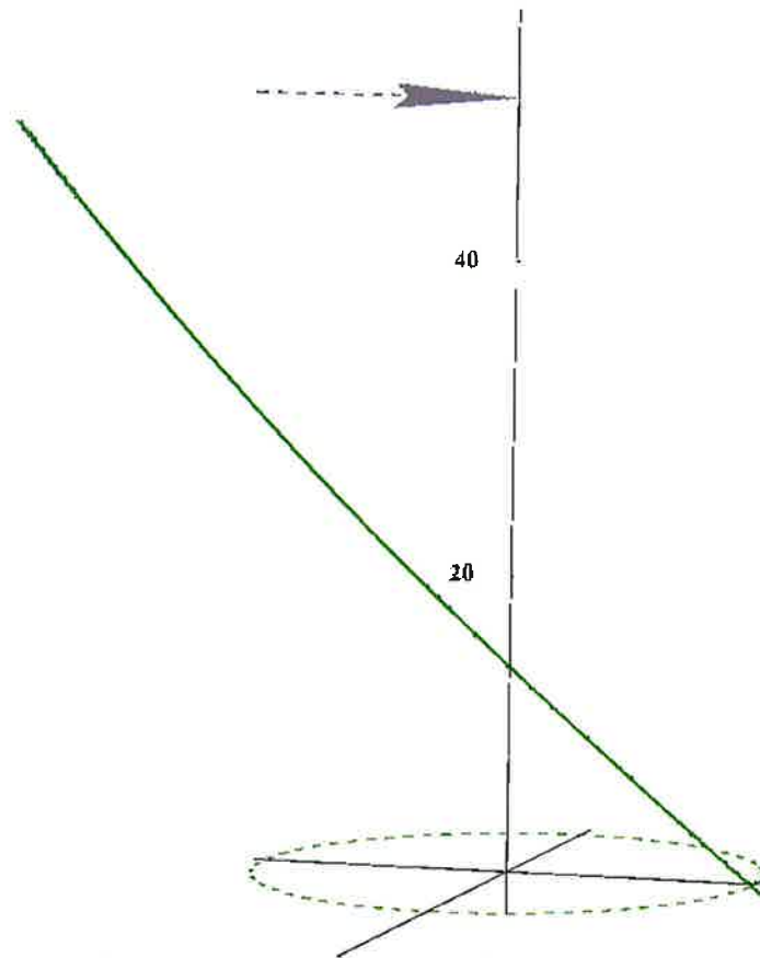
Abbildung 2: Flugbahn unter den gegebenen Randbedingungen – Eisobjekt Würfel (E-82, 78,0m Nabhöhe)
