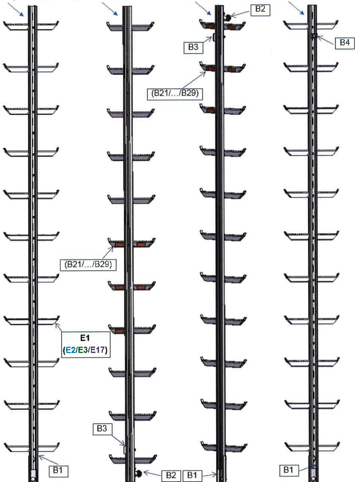
Fig. 2-3, Oberbaugruppen
