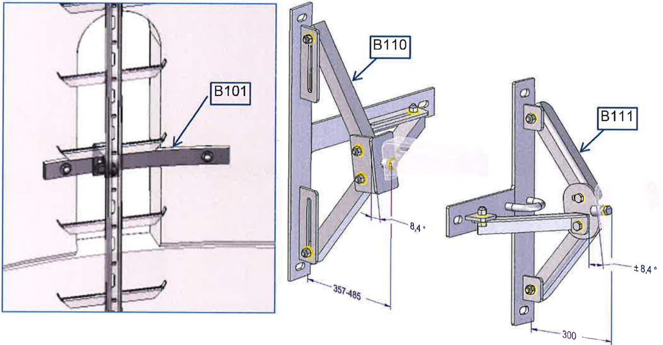
Fig. 2-17, Sonderhalter
