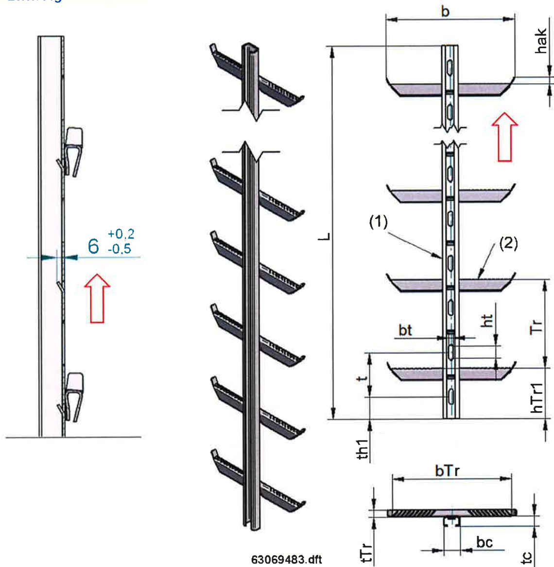
Fig. 2-7, LMB-Steigleiter
