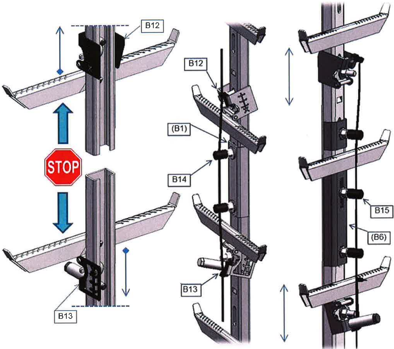
Fig. 2-11, LMB-Sperrklinke
