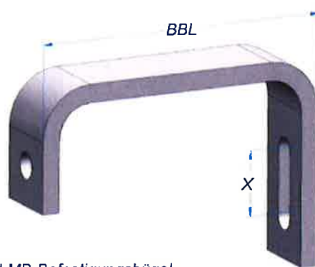
Fig. 2-16, LMB-Befestigungsbügel
