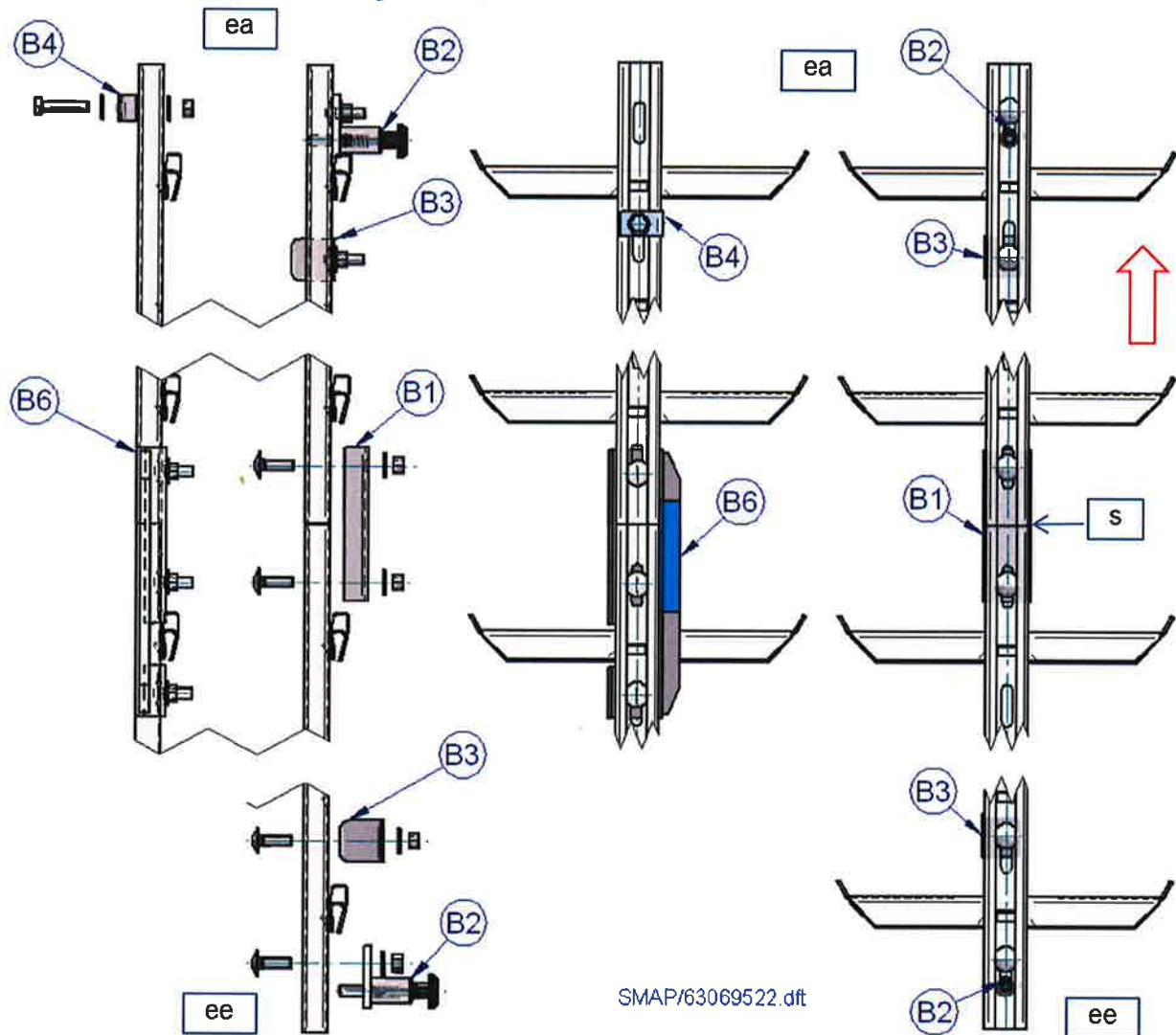
Fig. 2-8, LMB-Steigleiter
