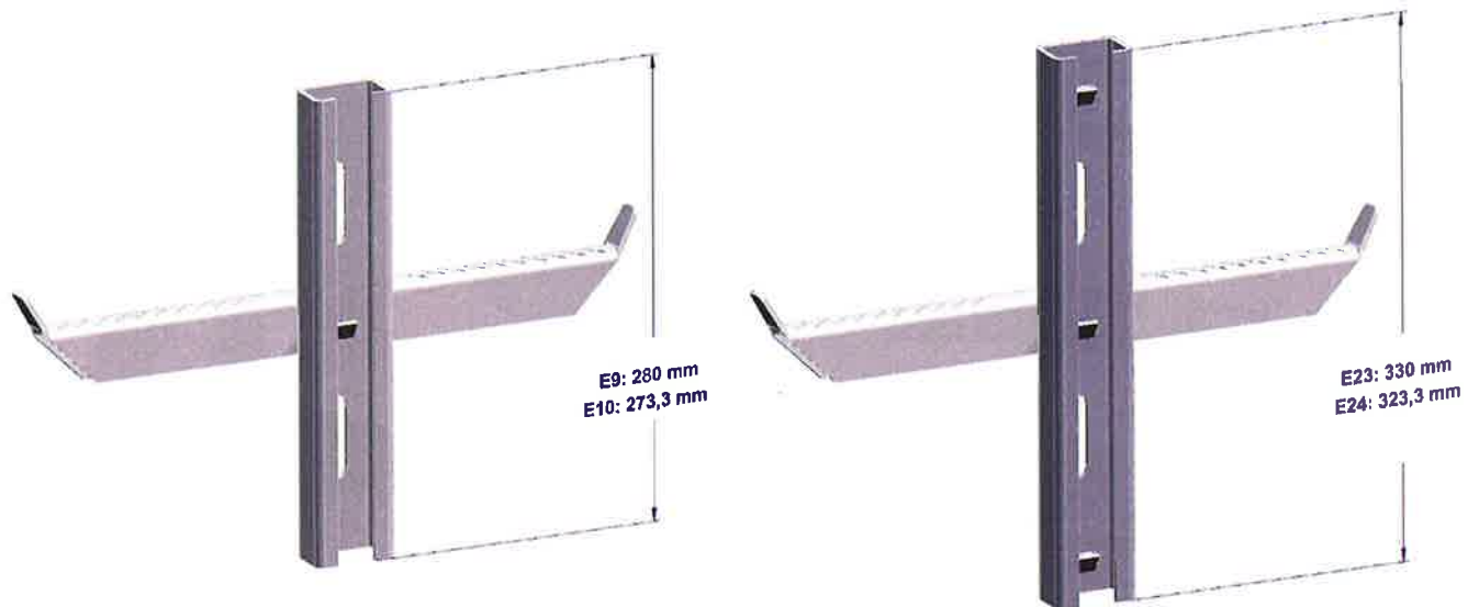
Fig. 2-20 LMB-Zwischensegmente
