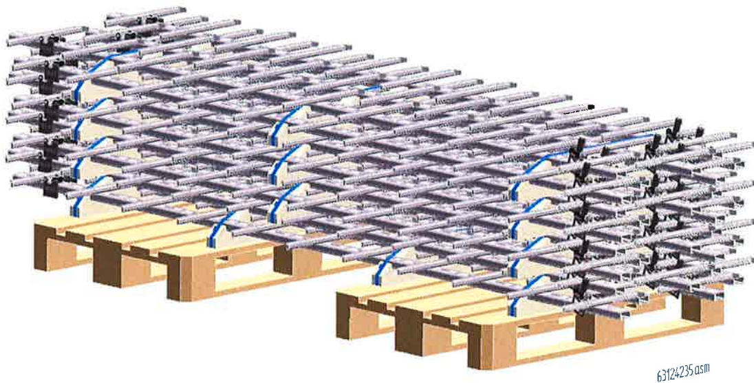
Fig. 2-4, LMB-Vormontage
