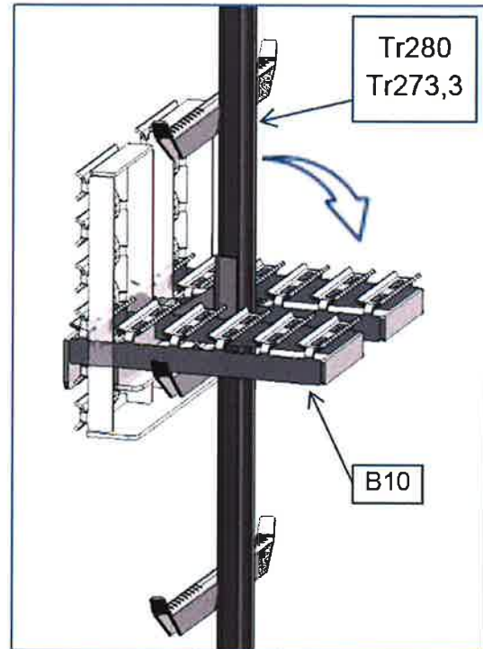
Fig. 2-19, LMB-Ruhepodest
