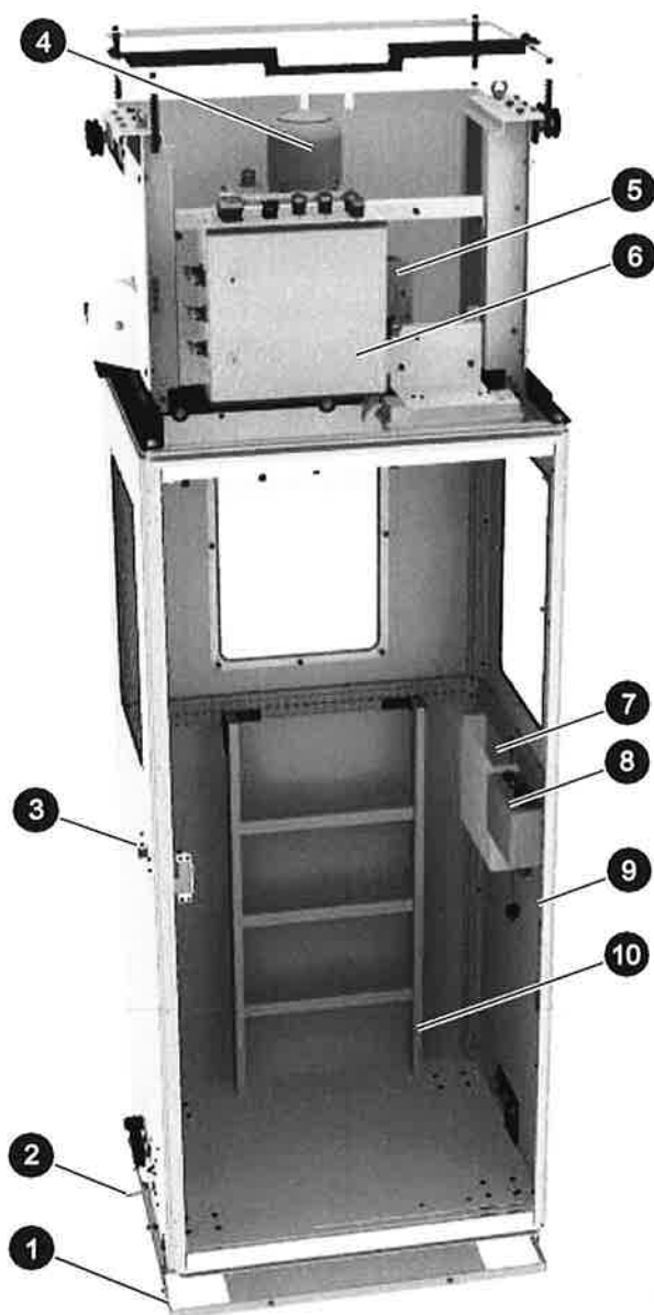
Abb. 2: Fahrkorb (innen)
