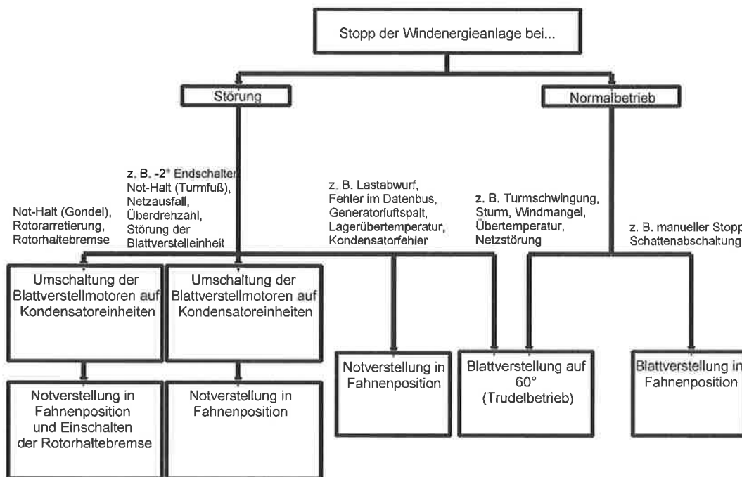
Abb. 5: Übersicht Windenergieanlagenstopp
