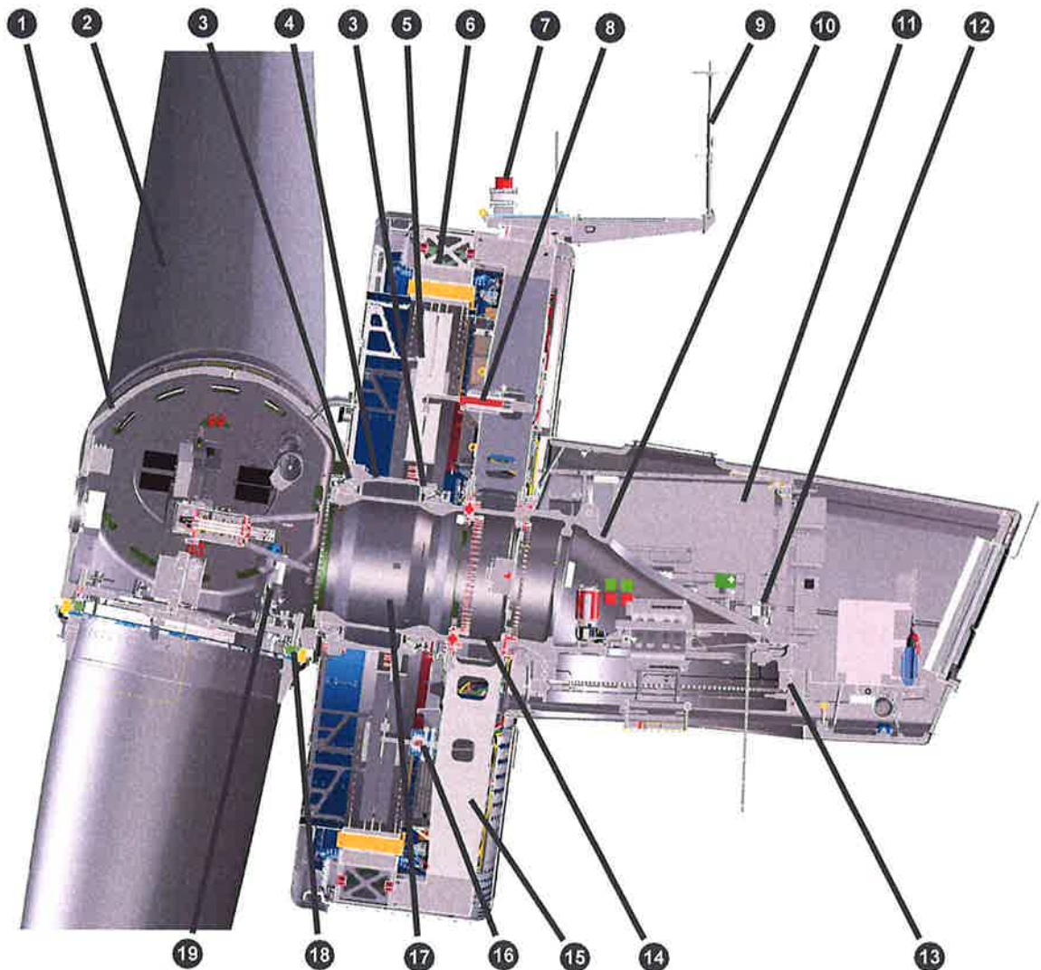
Abb. 2: Gondelschnitt
