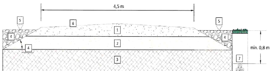
Abb. 16 Beispielhafter Aufbau der Zuwegung
