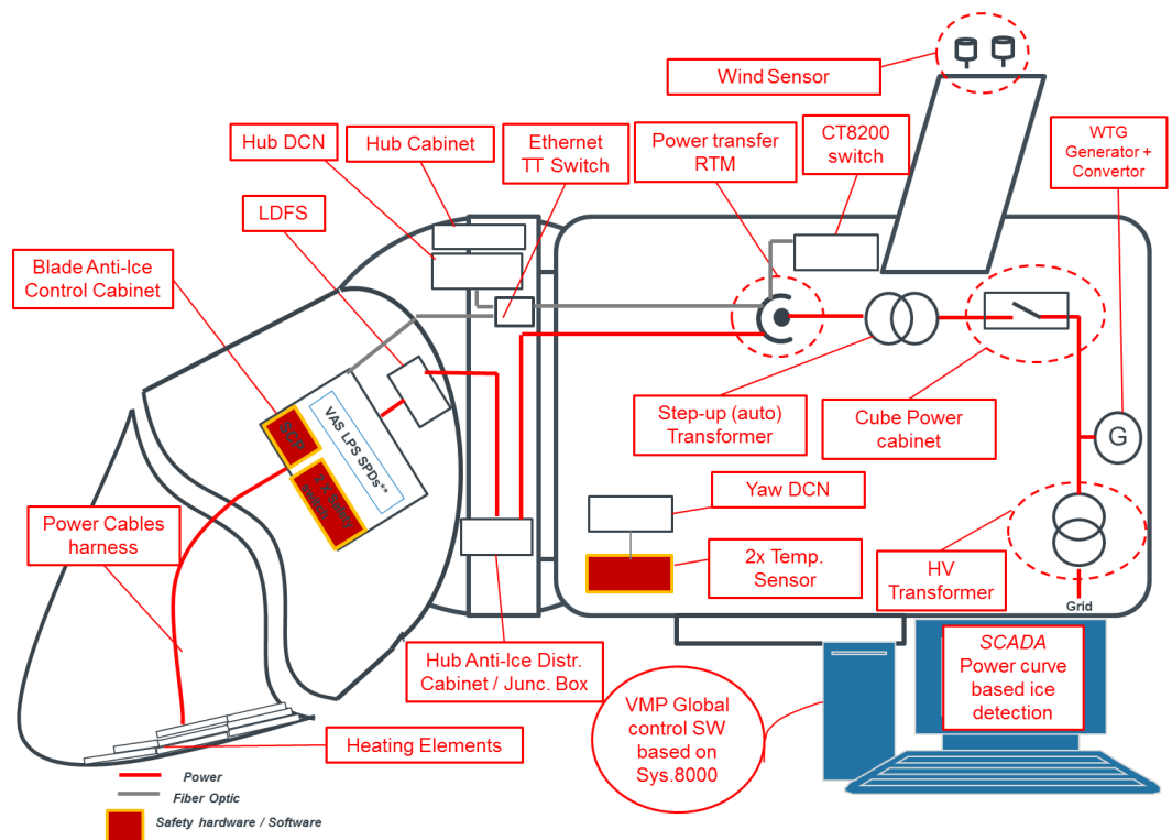
Abbildung 2. Schematische Darstellung der Integration des VAS in Windenergieanlagen
