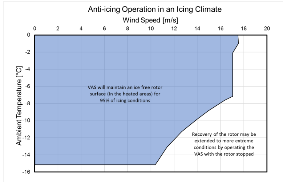
Abbildung 5. Beispiel Klimatische Abhängigkeit der VAS-Leistungsgrenze für 95 % aller Vereisungsbedingungen an einem Standort mit starkem Eisverlust in nordischen Ländern.
