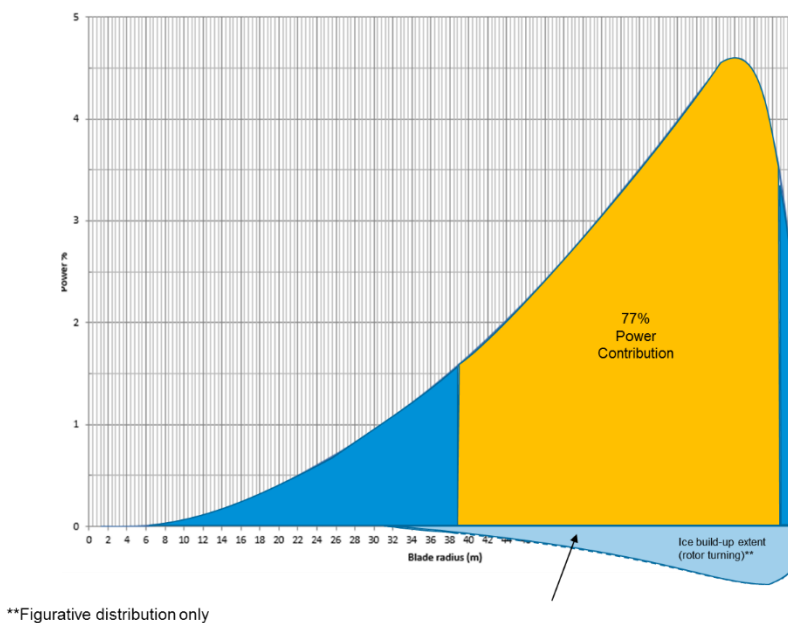
Abbildung 4 Beispielhafte Darstellung der Eisbildung, aerodynamischer Beitrag und Vereisungsschutzfläche eines VAS-Blattes. Die VAS-Varianten haben etwas unterschiedliche Bereiche.
