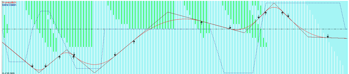
Bild 2: räumliche Linienführung Hinweg (gestrichelt blau: Krümmungsband; rot: Gradiente; links: -0+135)
