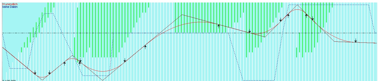
Bild 3: räumliche Linienführung Rückweg (gestrichelt blau: Krümmungsband; rot: Gradiente; links: -0+135)
