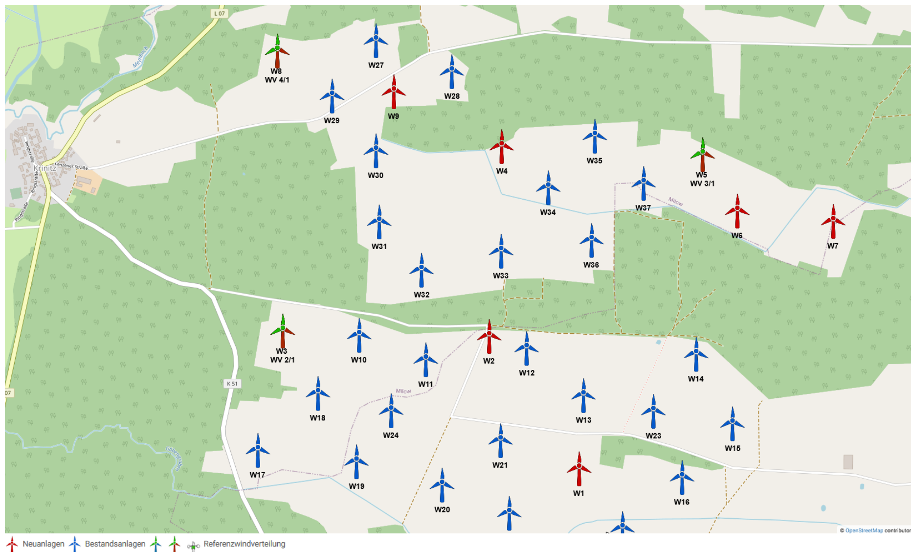
Abbildung 2.2: Zu untersuchende Windparkkonfiguration (Detail); Kartenmaterial: [19.1, 19.2]
