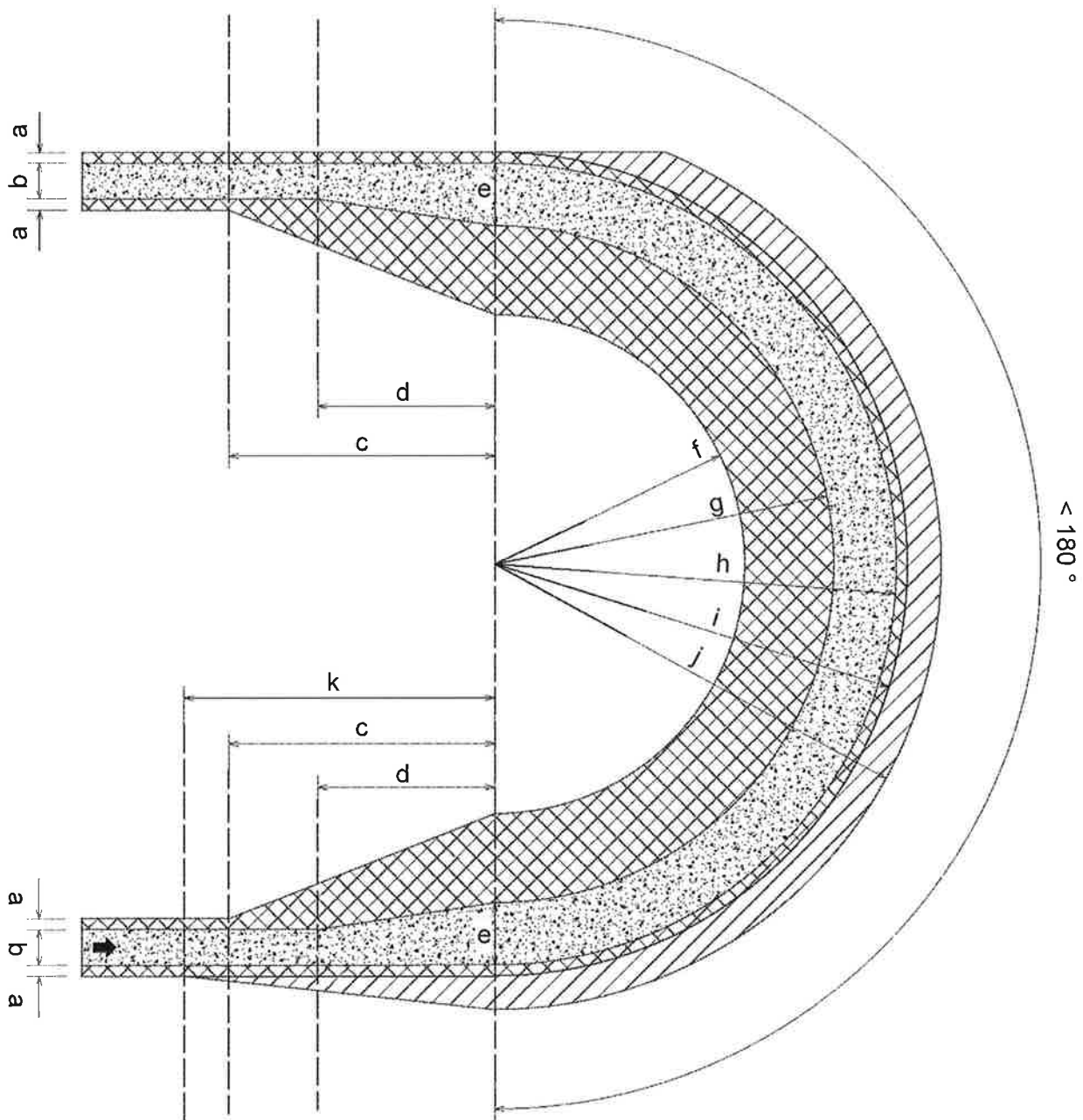
Abb. 3: 180-Grad-Kurve (Konstruktionsschema)
