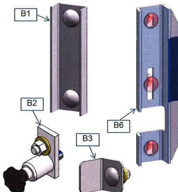
Fig. 2-9, LMB-Steigleiter
