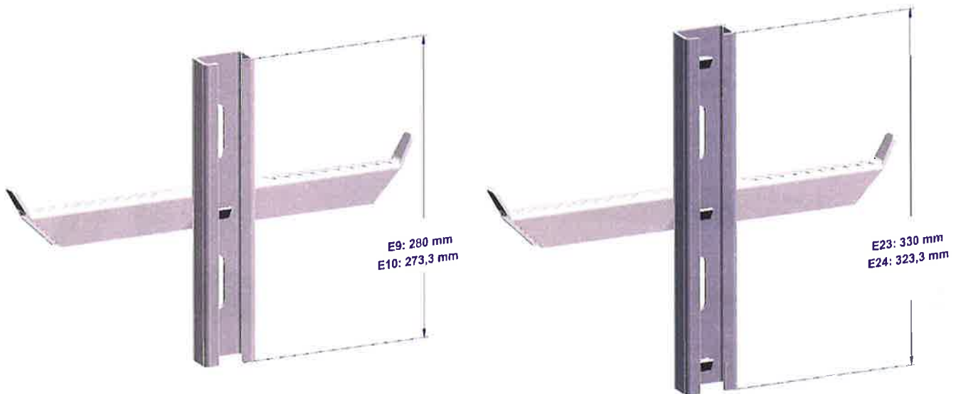
Fig. 2-20 LMB-Zwischensegmente
