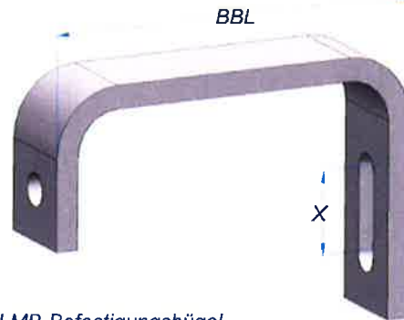
Fig. 2-16, LMB-Befestigungsbügel
