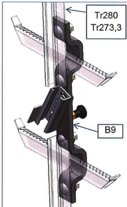
Fig. 2-18, LMB-Ausstiegsvorrichtung
