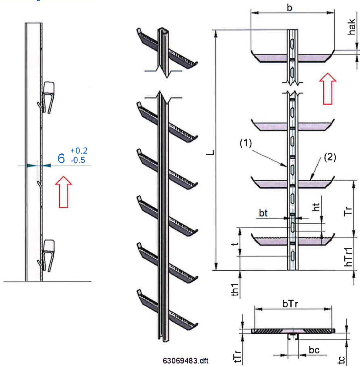
Fig. 2-7, LMB-Steigleiter
