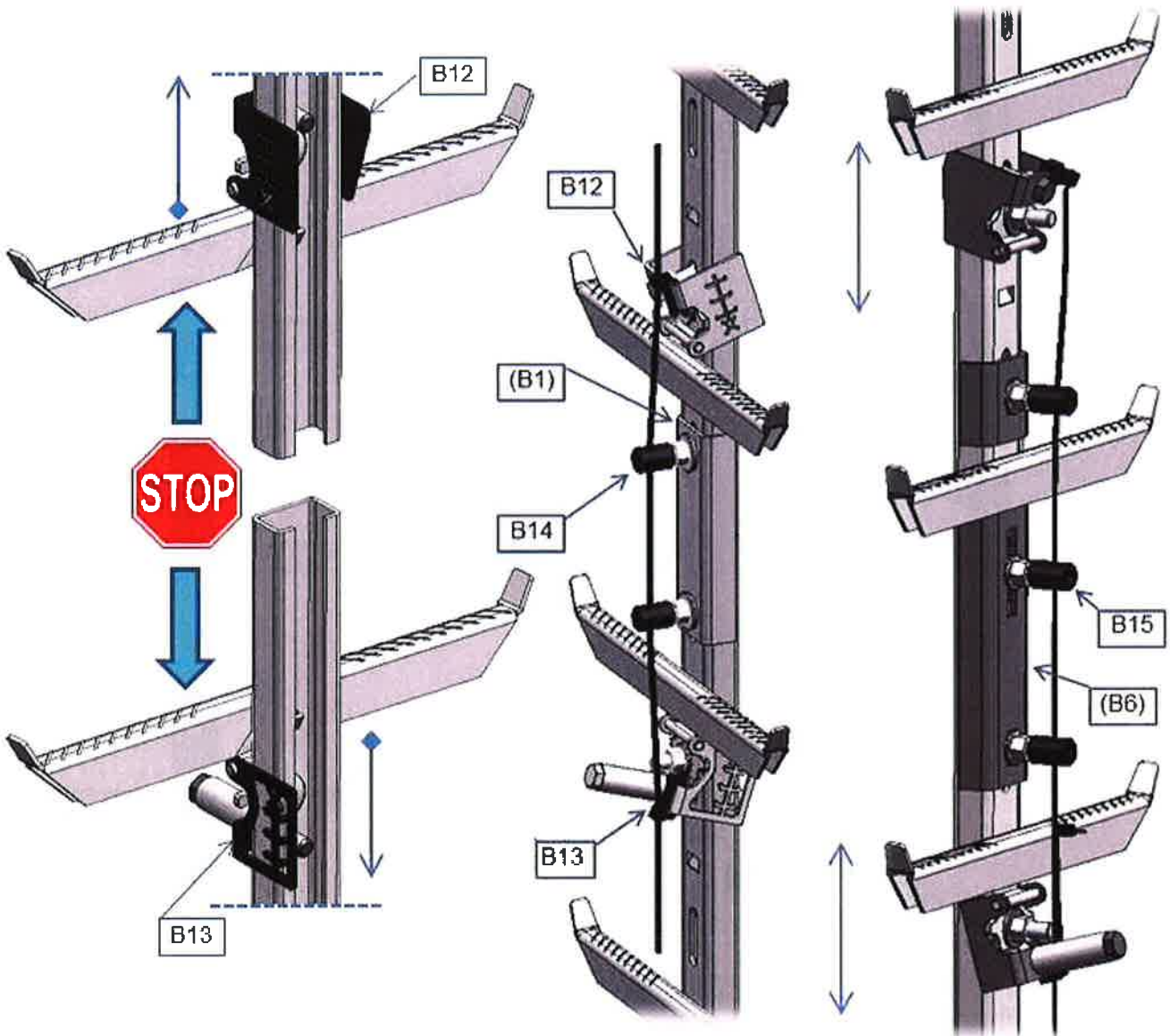
Fig. 2-11, LMB-Sperrklinke
