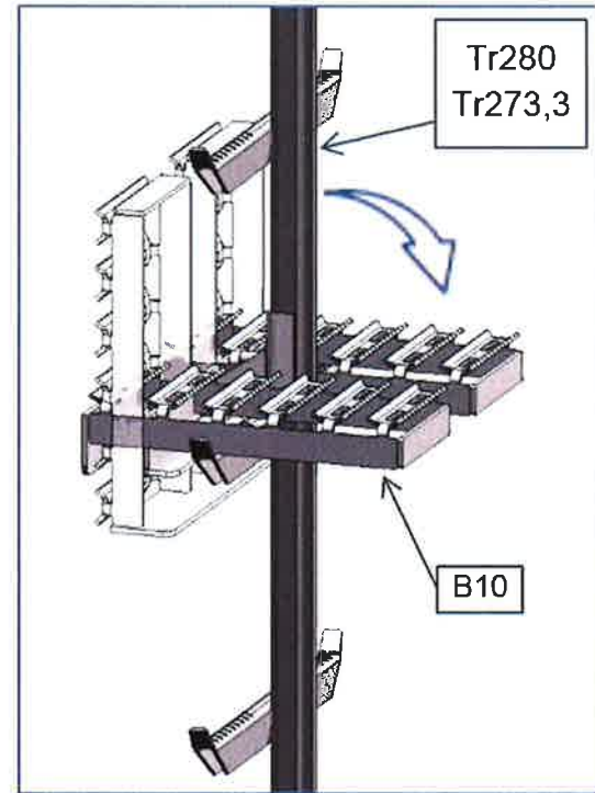
Fig. 2-19, LMB-Ruhepodest
