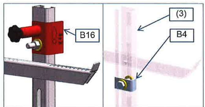
Fig. 2-10, LMB-Steigleiter
