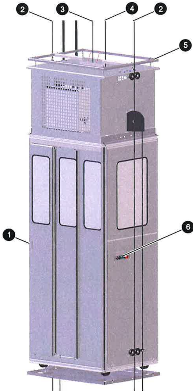
Abb. 1: Fahrkorb (außen)
