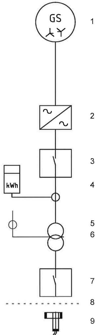
Abb. 1: Prinzipschaltbild ENERCON WEA Standard 1
