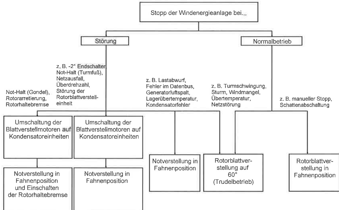
Abb. 5: Übersicht Windenergieanlagenstopp
