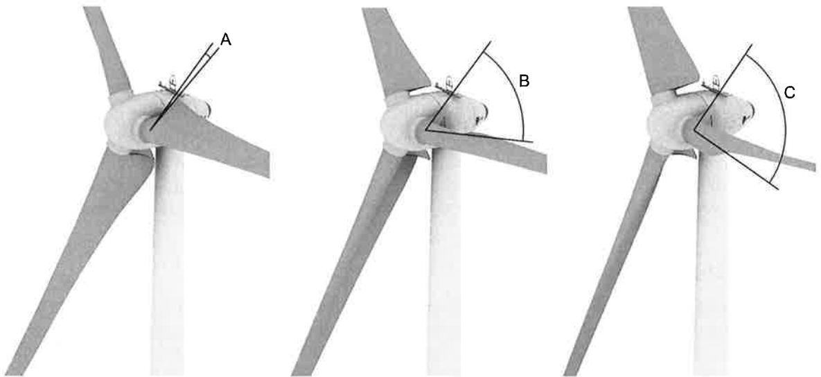
Abb. 4: Besondere Rotorblattstellungen
