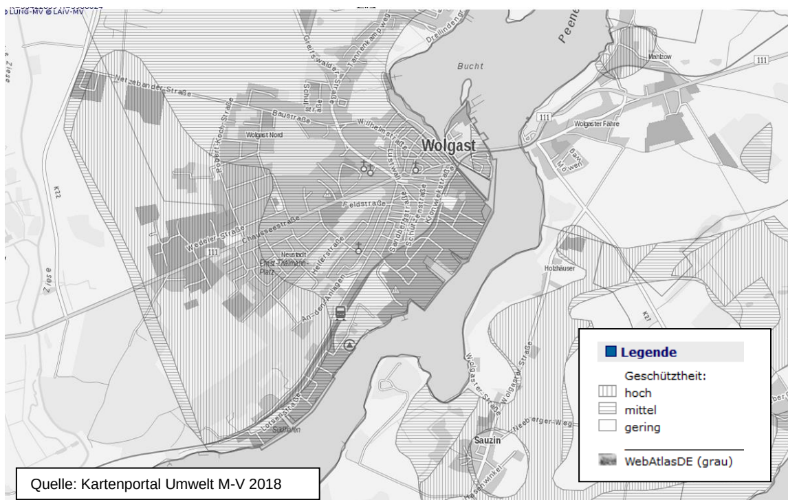
Abbildung 3: Gebiete mit geringem Grundwasserflurabstand
