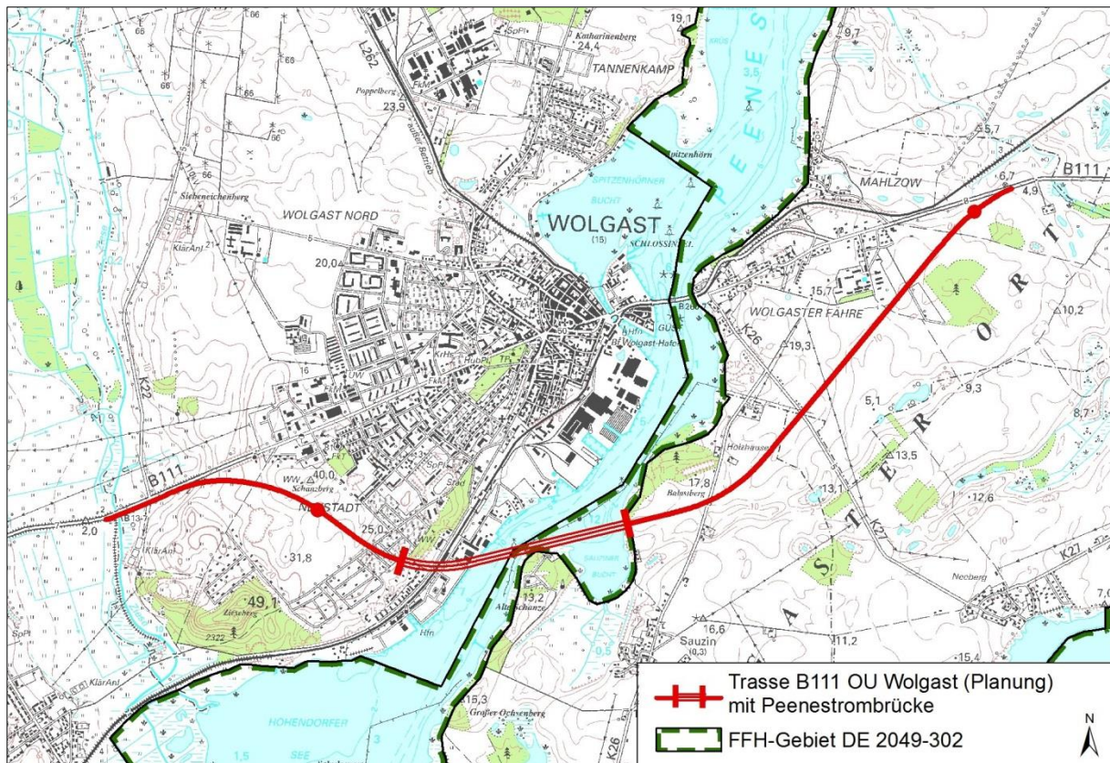
Abb. 2: Trassierung der geplanten B 111 OU Wolgast und Lage im FFH-Gebiet
