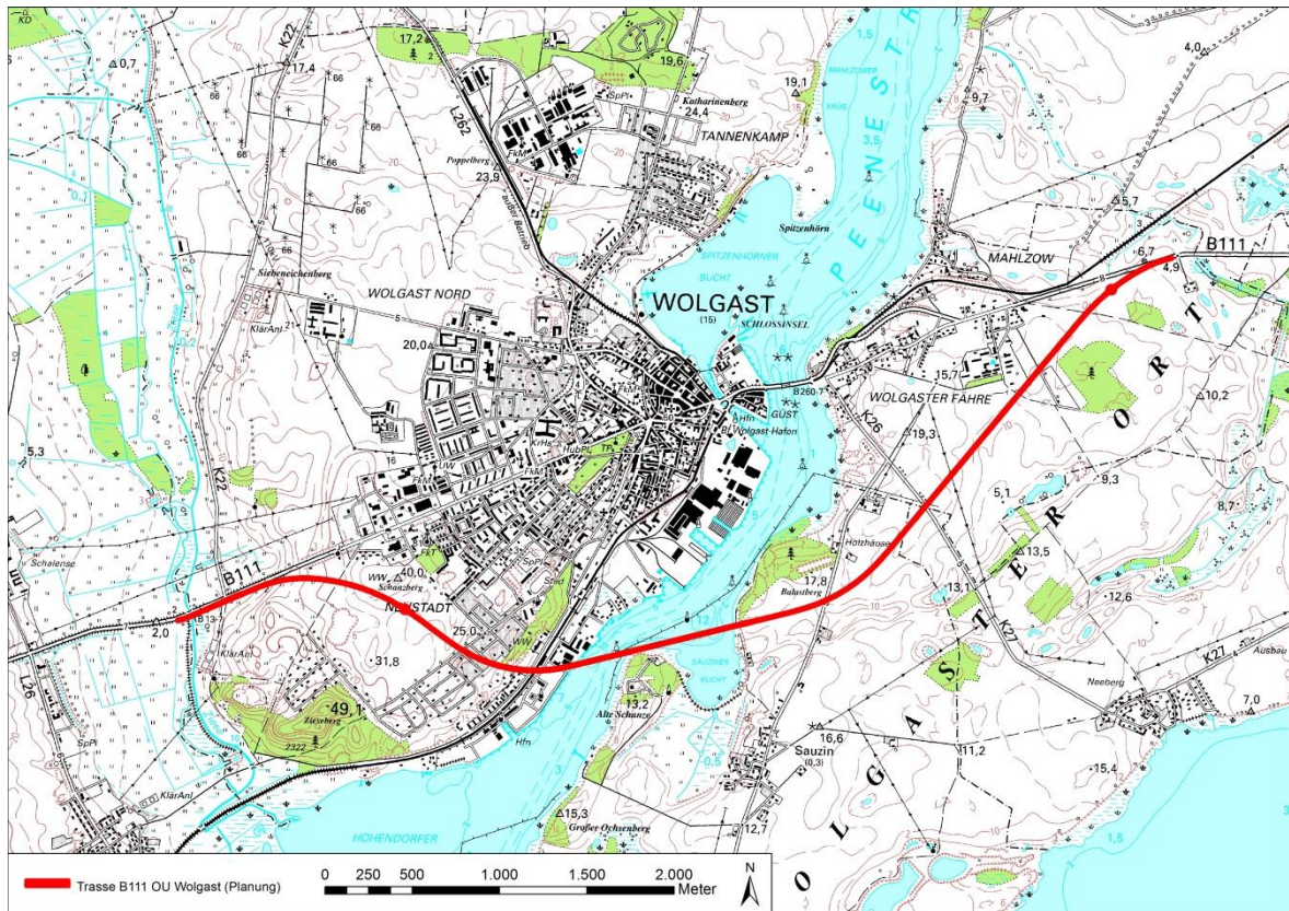
Abb. 1: Trassierung der geplanten B 111 OU Wolgast
